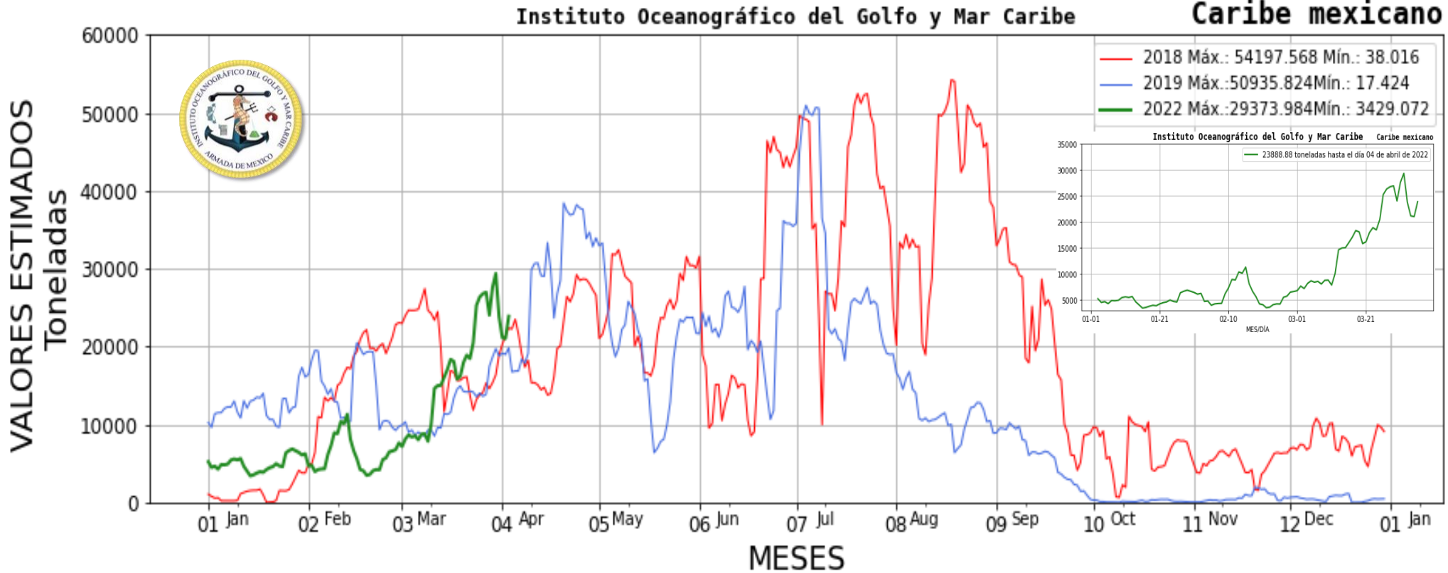
Figura 2.- Valores estimados de la cantidad de sargazo en el Caribe Mexicano. Gráfico comparativo de los años 2018, 2019 y 2022 (gráfico mayor) y valores estimados del 01 de enero al 04 de abril del presente año (gráfico superior derecha) obtenidos a partir de datos de la USF.
