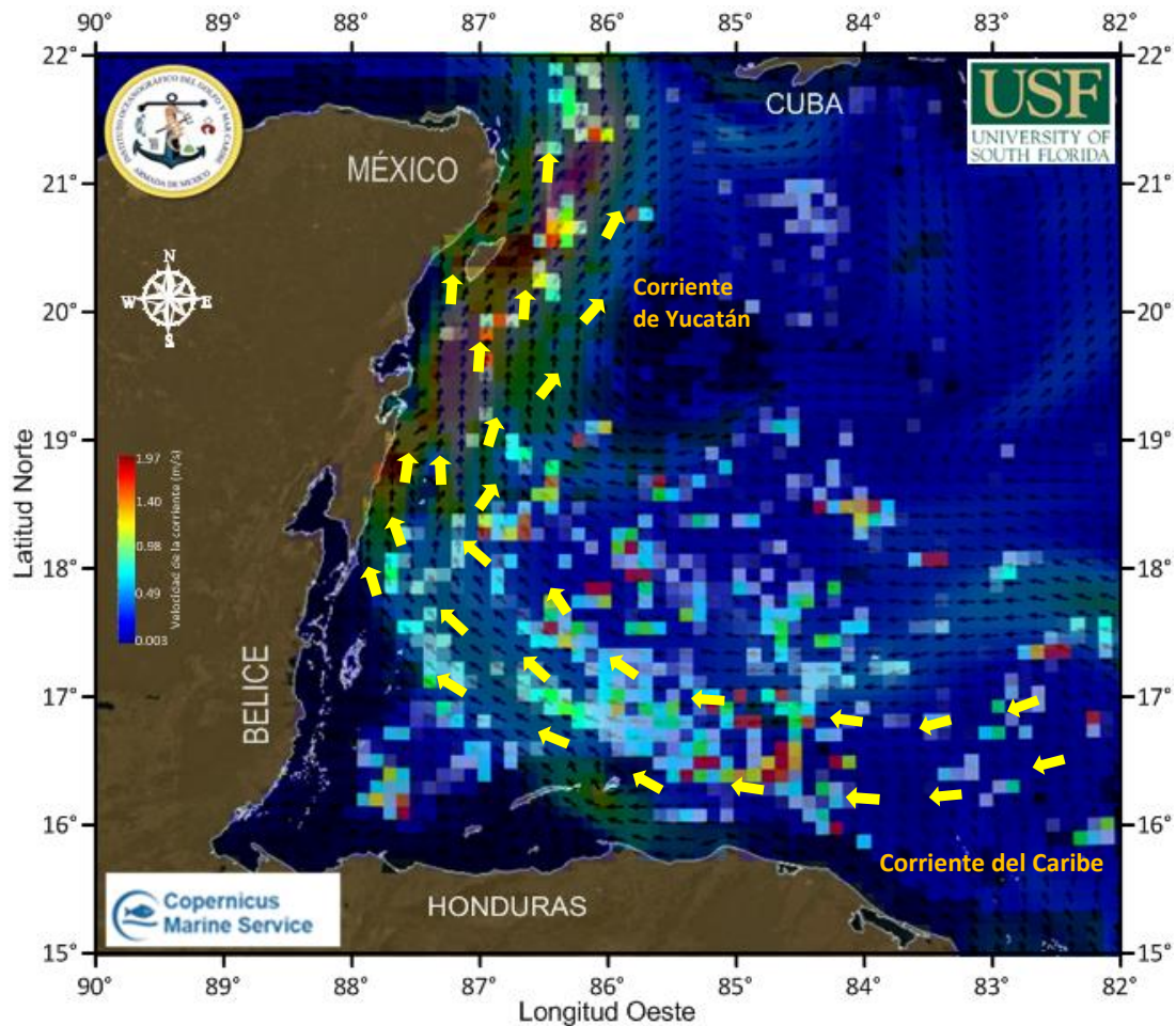
Figura 1.- Cobertura algal (04 de abril) v modelación de corrientes superficiales (05 de abril).
