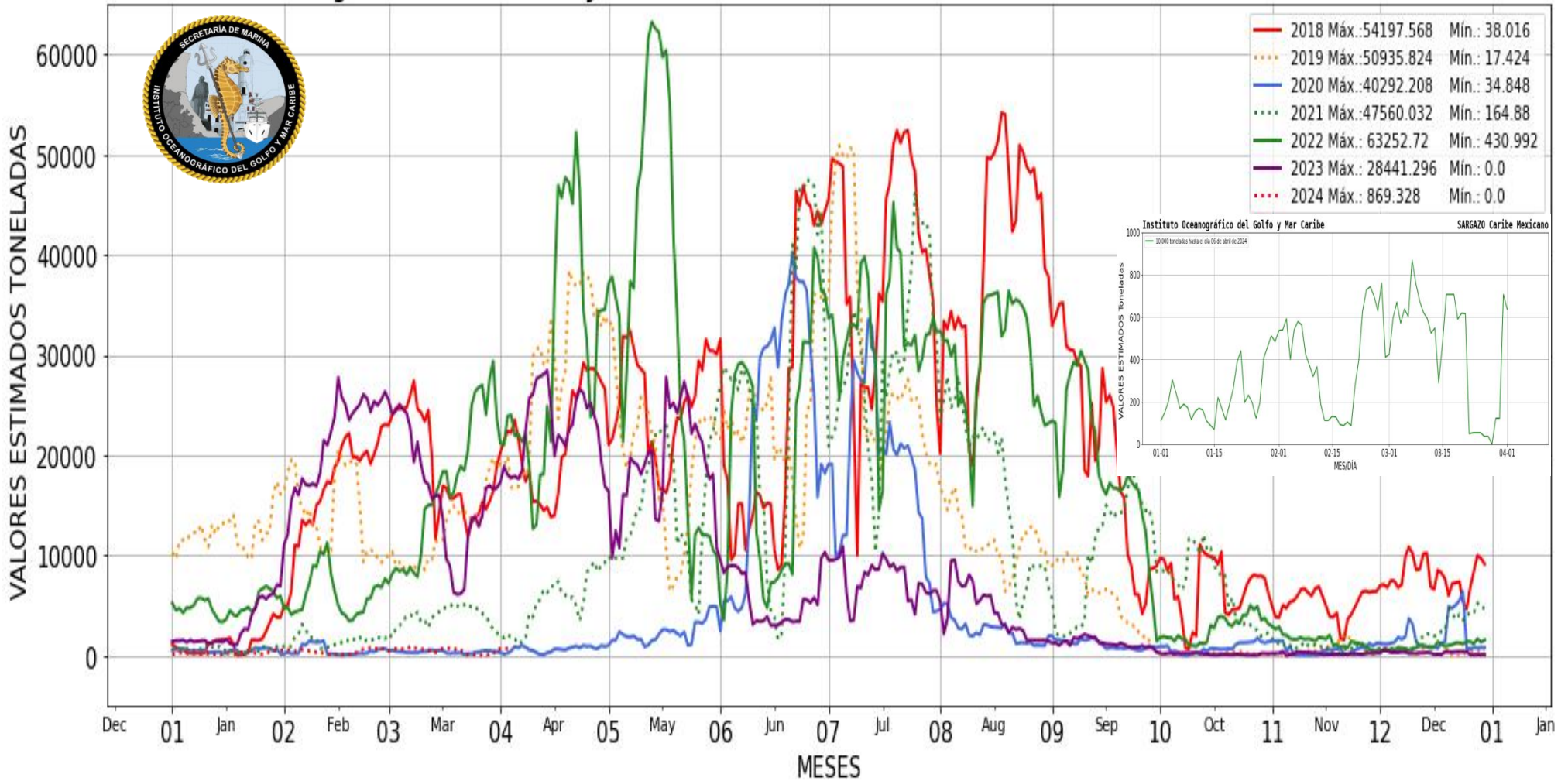
Figura 2.- Densidad de sargazo calculada a partir de la media acumulada. Gráfico comparativo de los años 2018-2024 (gráfico mayor) y valores estimados del 01 de enero al 06 de abril del presente año (gráfico superior derecho) obtenidos a partir de datos de la USF.
