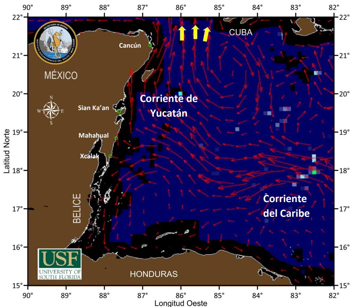
Figura 1.- Cobertura algal (06 de abril) y la modelación de corrientes superficiales (07 de abril), obtenidos a partir de datos de la USF.
