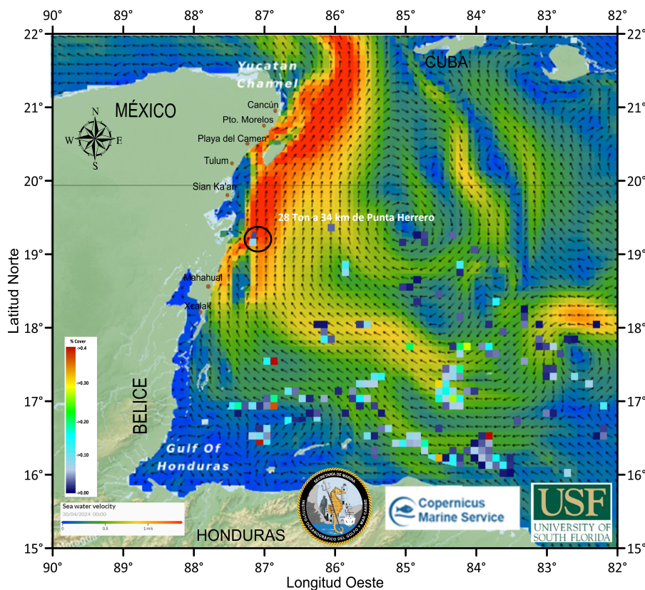
Figura 2.- Cobertura algal ( 29 de abril ) y la modelación de corrientes superficiales ( 30 de abril ), obtenidos a partir de datos de la USF.
