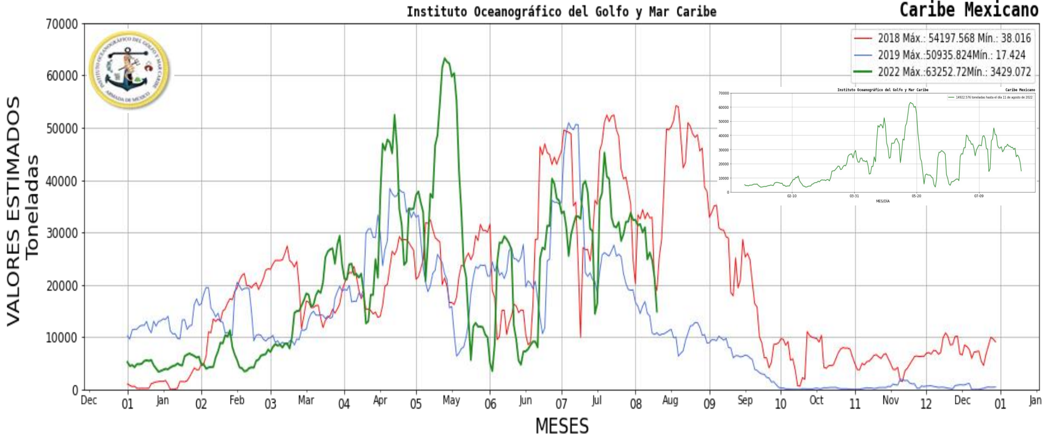
Figura 2.- Valores estimados de la cantidad de sargazo en el Caribe Mexicano. Gráfico comparativo de los años 2018, 2019 y 2022 (gráfico mayor) y valores estimados del 01 de enero al 11 de agosto del presente año (gráfico superior derecha) obtenidos a partir de datos de la USF.
