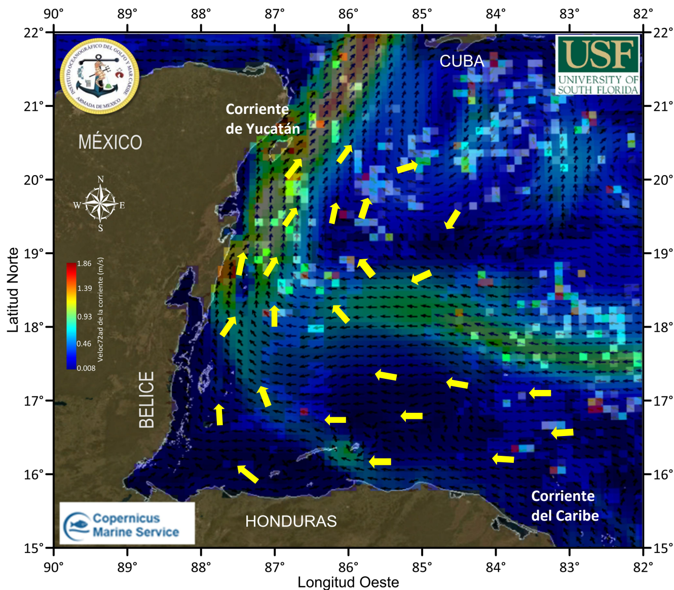
Figura 1.- Cobertura algal (11 de agosto) y modelación de corrientes superficiales (12 de agosto).
