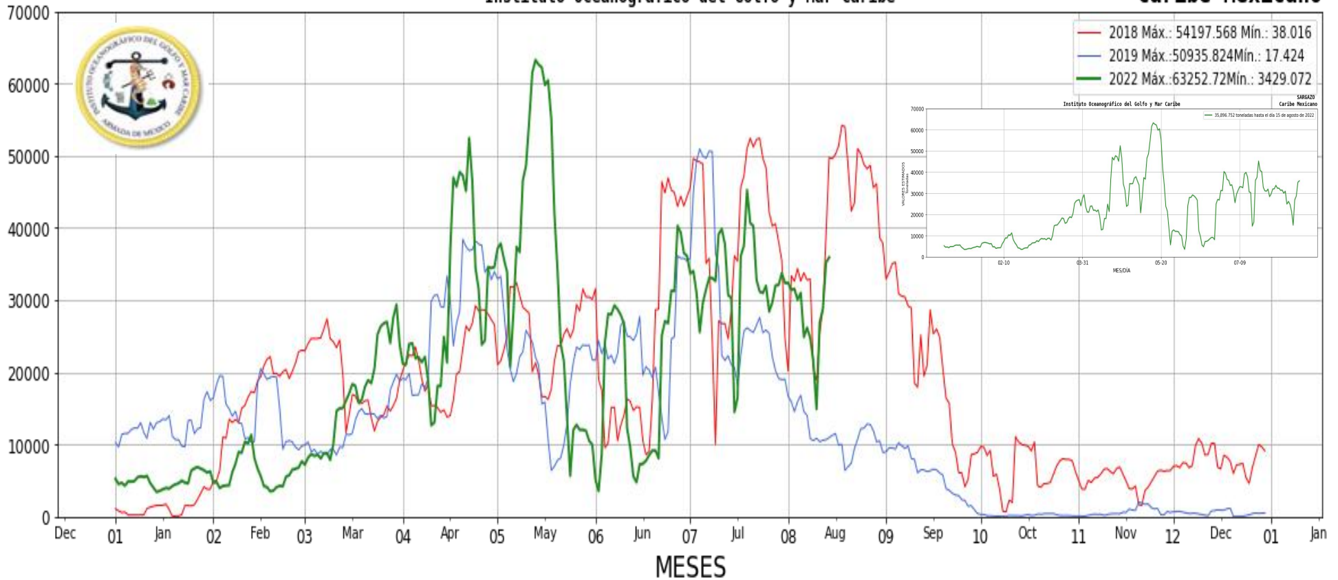
Figura 2.- Valores estimados de la cantidad de sargazo en el Caribe Mexicano. Gráfico comparativo de los años 2018, 2019 y 2022 (gráfico mayor) y valores estimados del 01 de enero al 15 de agosto del presente año (gráfico superior derecha) obtenidos a partir de datos de la USF.
