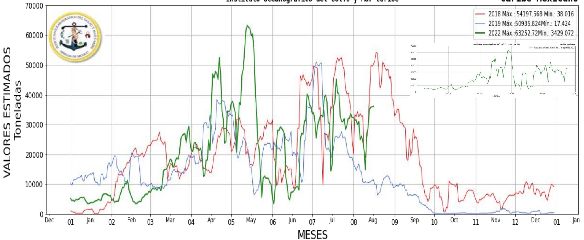
Figura 2.- Valores estimados de la cantidad de sargazo en el Caribe Mexicano. Gráfico comparativo de los años 2018, 2019 y 2022 (gráfico mayor) y valores estimados del 01 de enero al 17 de agosto del presente año (gráfico superior derecha) obtenidos a partir de datos de la USF.
