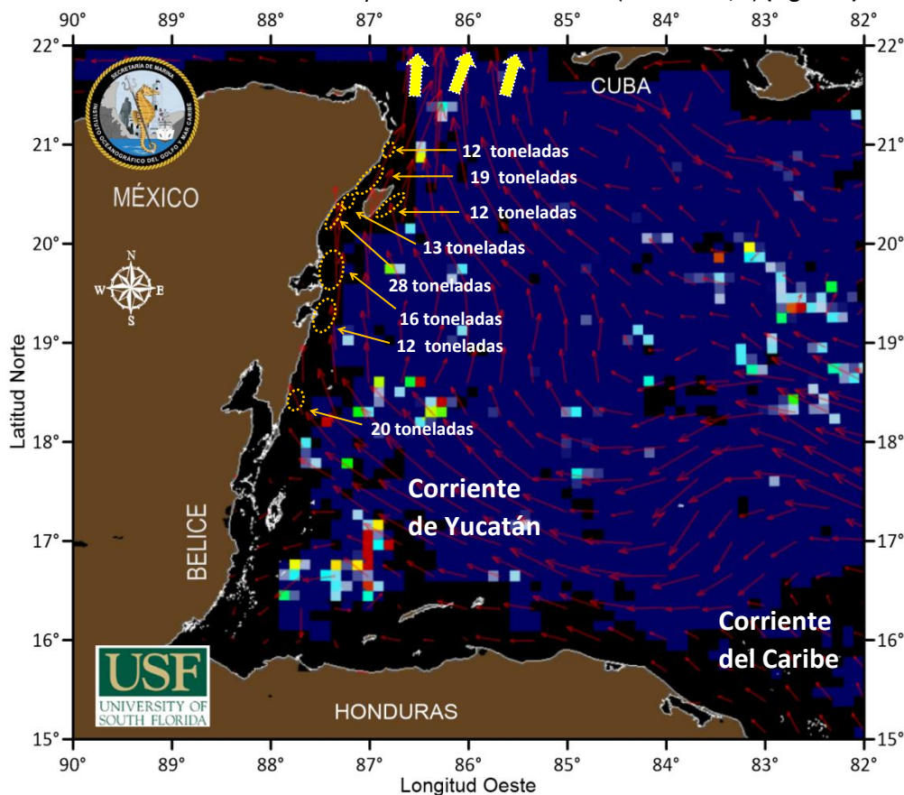
Figura 1.- Cobertura algal (31 de julio) y la modelación de corrientes superficiales (01 de agosto), obtenidos a partir de datos de la USF.
