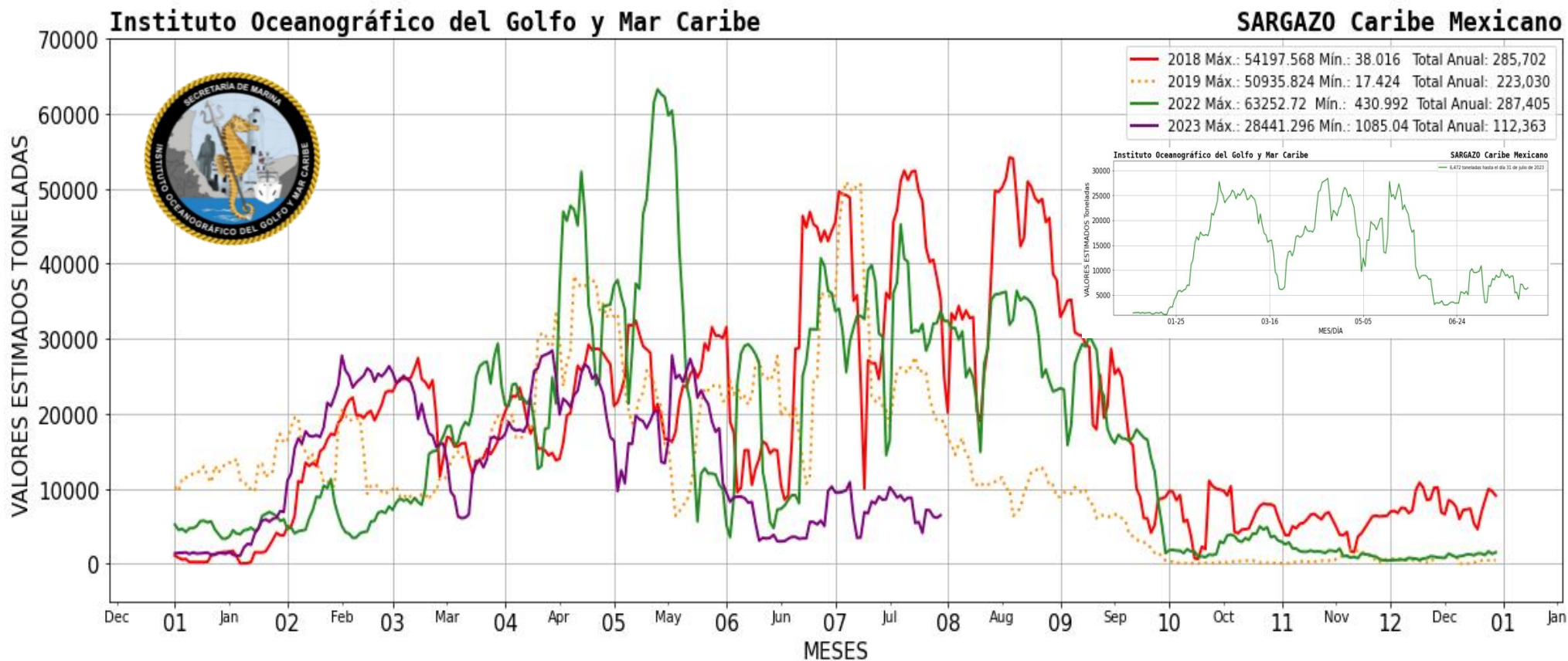
Figura 2.- Presencia aproximada de sargazo en el Caribe Mexicano. Gráfico comparativo de los años 2018, 2019, 2022 y 2023 (gráfico mayor) y valores estimados del 01 de enero al 31 de julio del presente año (gráfico superior derecho) obtenidos a partir de datos de la USF.
