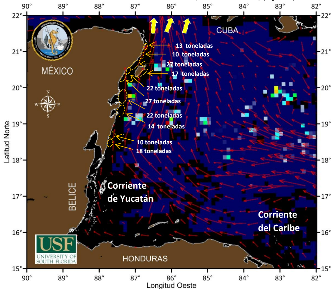
Figura 1.- Cobertura algal (04 de agosto) y la modelación de corrientes superficiales (05 de agosto), obtenidos a partir de datos de la USF.
