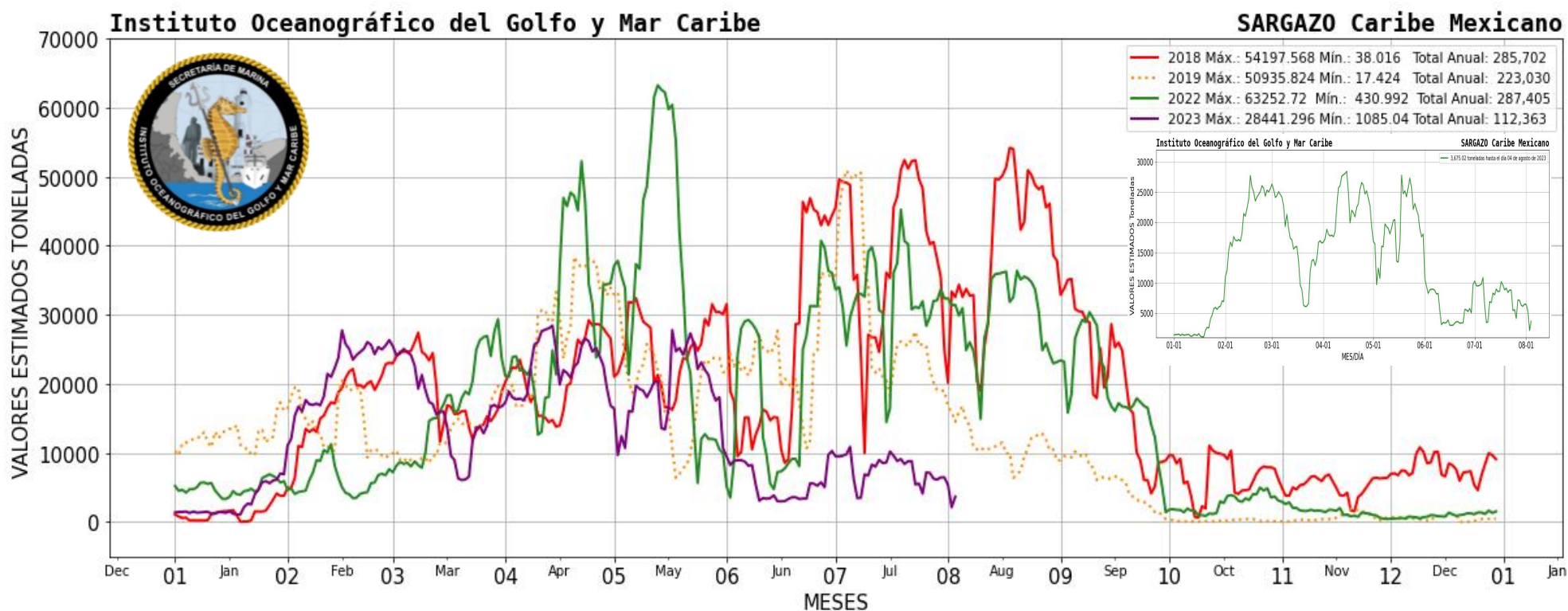
Figura 2.- Presencia aproximada de sargazo en el Caribe Mexicano. Gráfico comparativo de los años 2018, 2019, 2022 y 2023 (gráfico mayor) y valores estimados del 01 de enero al 04 de agosto del presente año (gráfico superior derecho) obtenidos a partir de datos de la USF.
