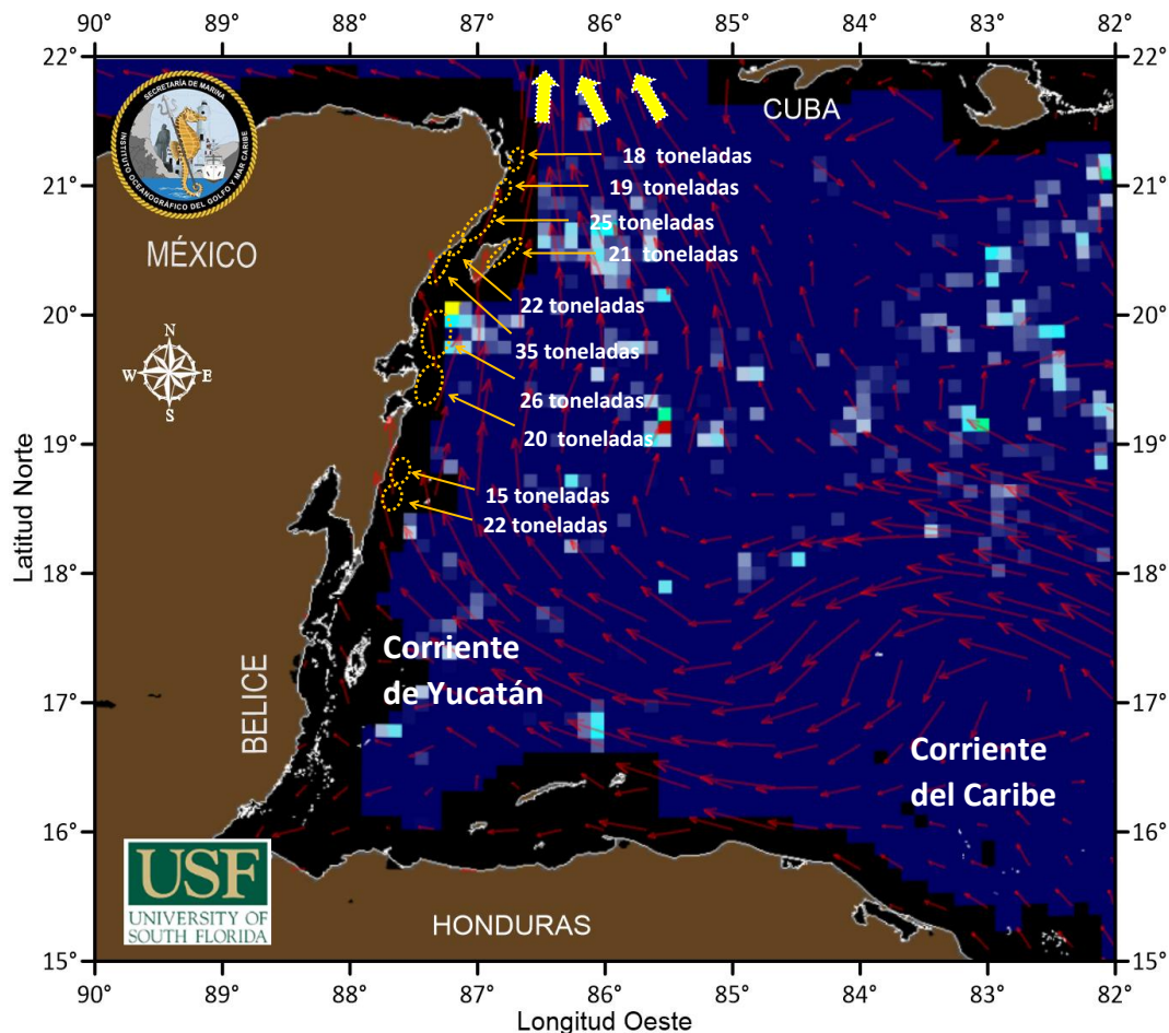
Figura 1.- Cobertura algal (08 de agosto) y la modelación de corrientes superficiales (09 de agosto), obtenidos a partir de datos de la USF.
