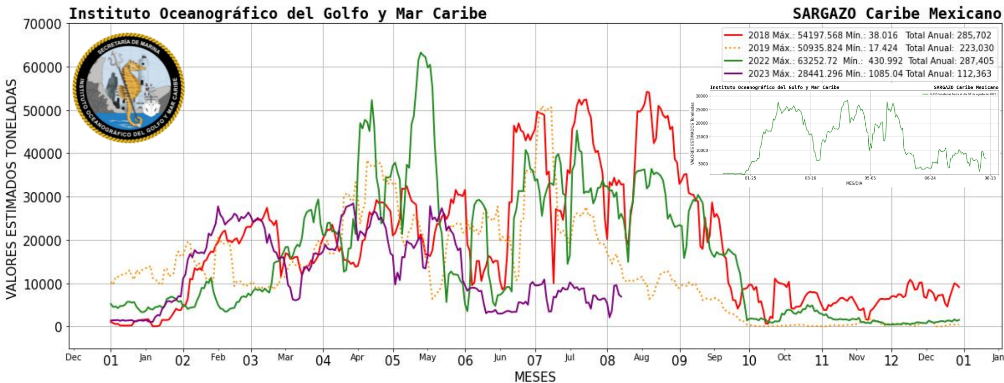
Figura 2.- Presencia aproximada de sargazo en el Caribe Mexicano. Gráfico comparativo de los años 2018, 2019, 2022 y 2023 (gráfico mayor) y valores estimados del 01 de enero al 08 de agosto del presente año (gráfico superior derecho) obtenidos a partir de datos de la USF.
