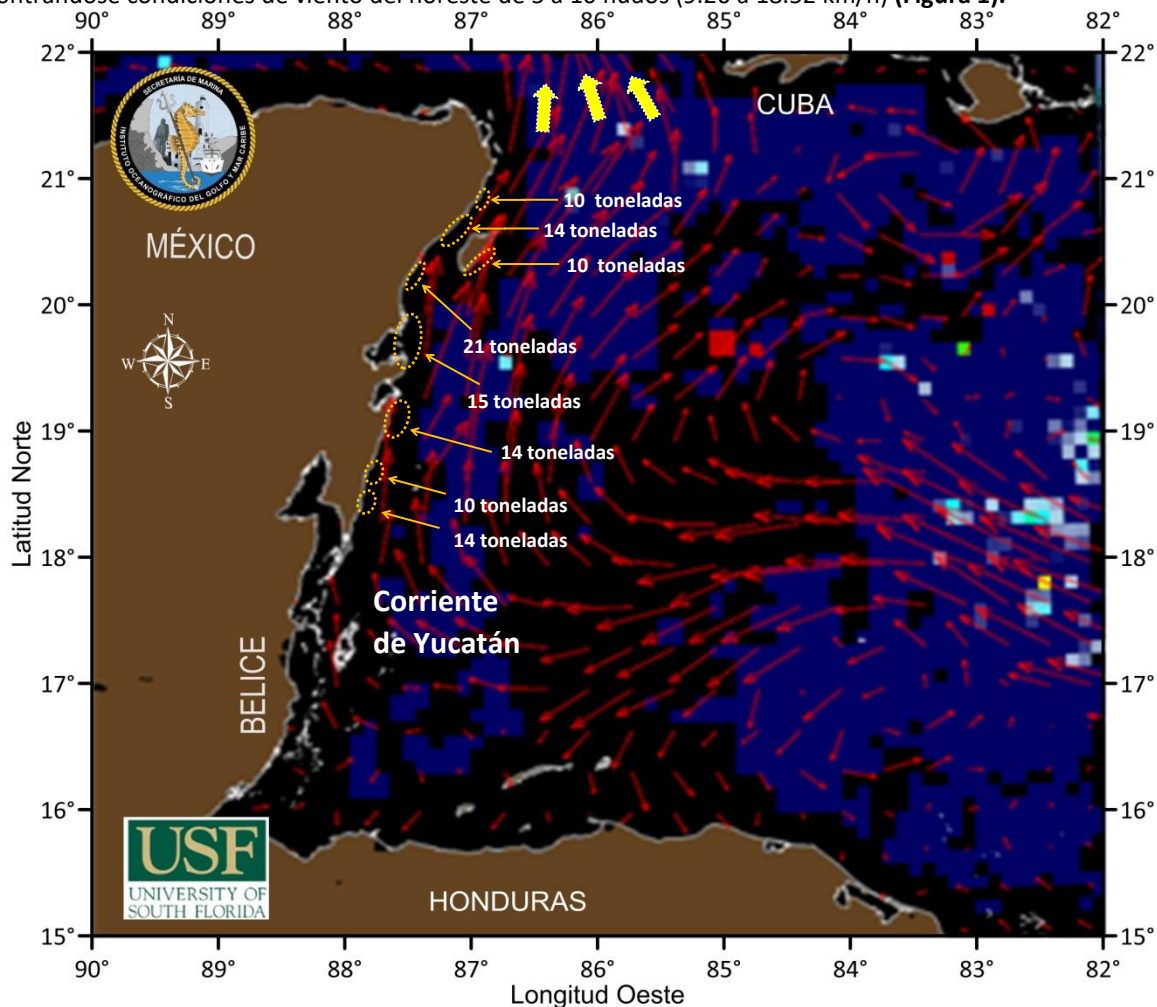
Figura 1.- Cobertura algal (20 de agosto) y la modelación de corrientes superficiales (21 de agosto), obtenidos a partir de datos de la USF.
