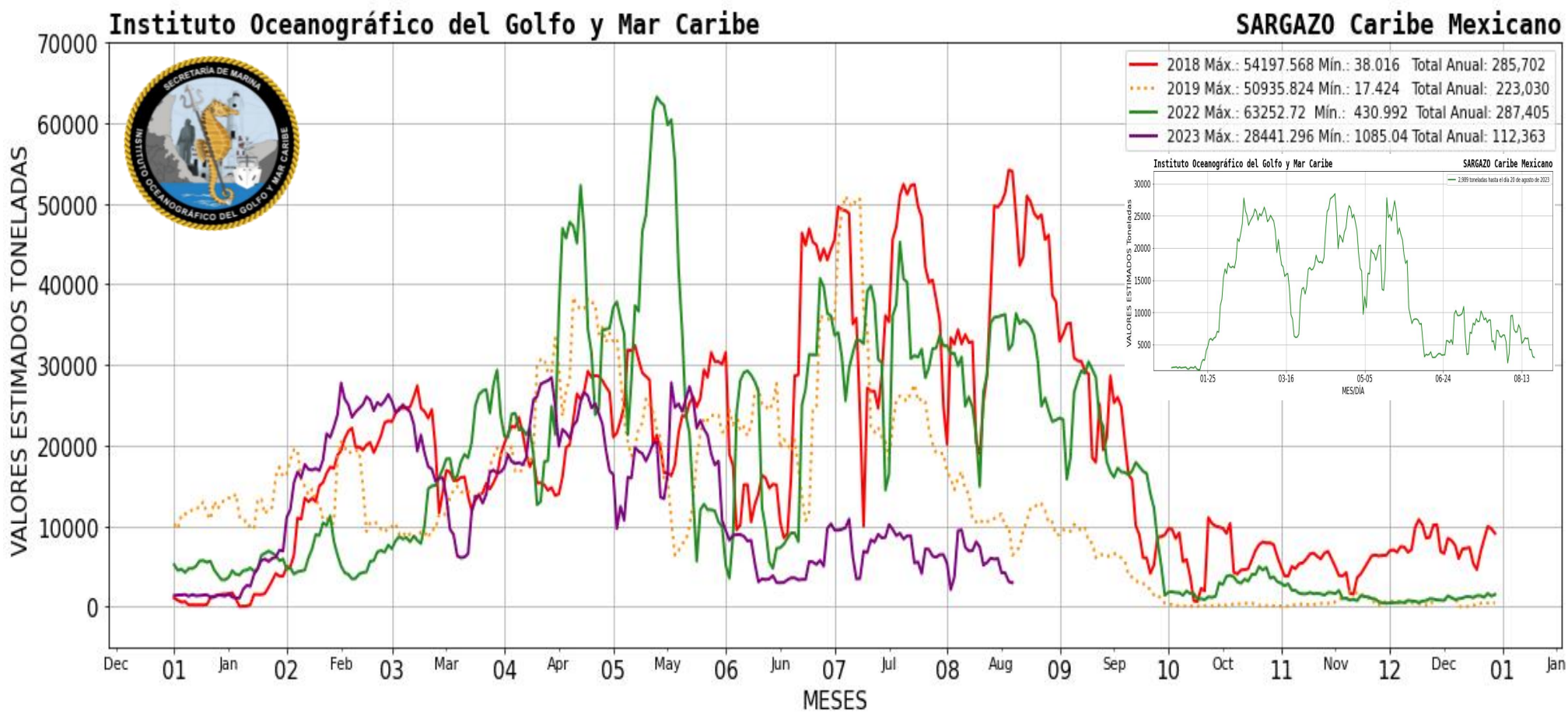
Figura 2.- Presencia aproximada de sargazo en el Caribe Mexicano. Gráfico comparativo de los años 2018, 2019, 2022 y 2023 (gráfico mayor) y valores estimados del 01 de enero al 20 de agosto del presente año (gráfico superior derecho) obtenidos a partir de datos de la USF.
