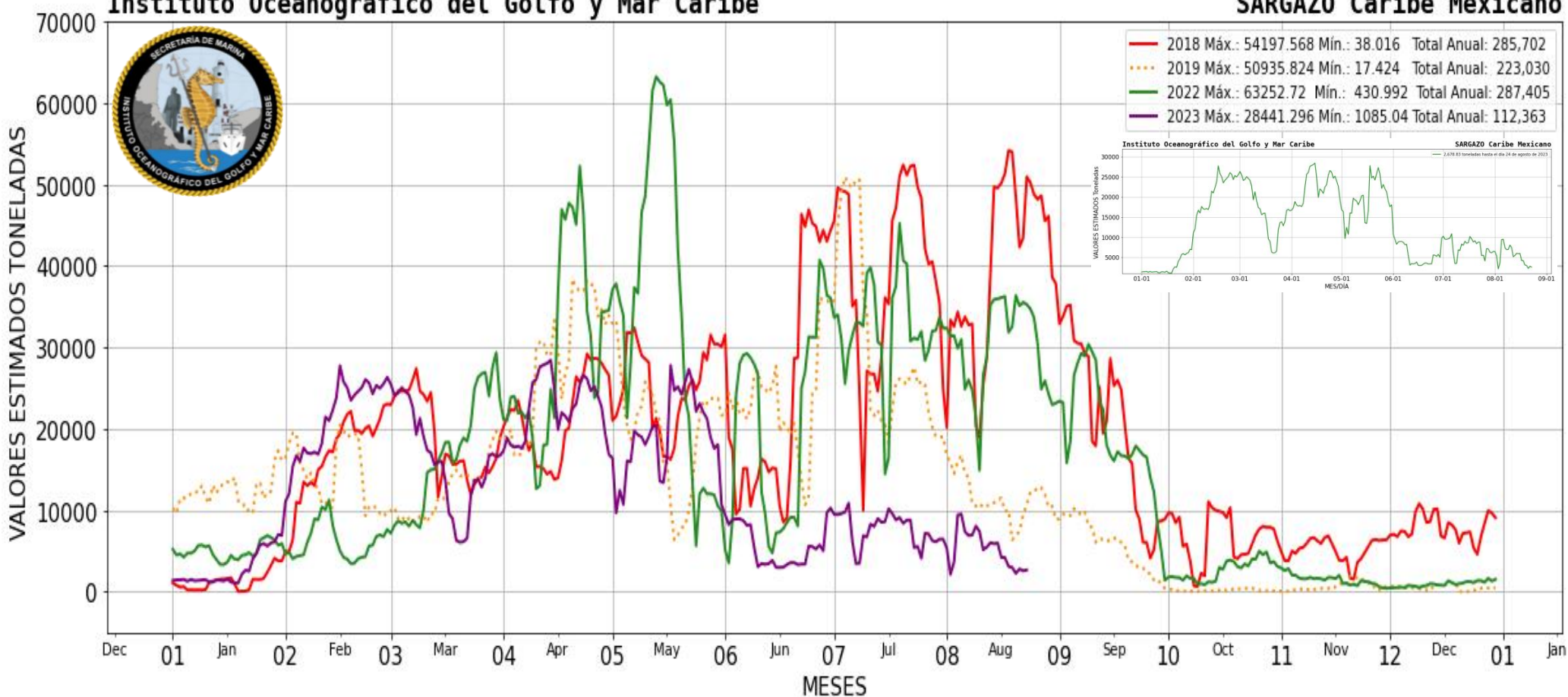
Figura 2.- Presencia aproximada de sargazo en el Caribe Mexicano. Gráfico comparativo de los años 2018, 2019, 2022 y 2023 (gráfico mayor) y valores estimados del 01 de enero al 24 de agosto del presente año (gráfico superior derecho) obtenidos a partir de datos de la USF.
