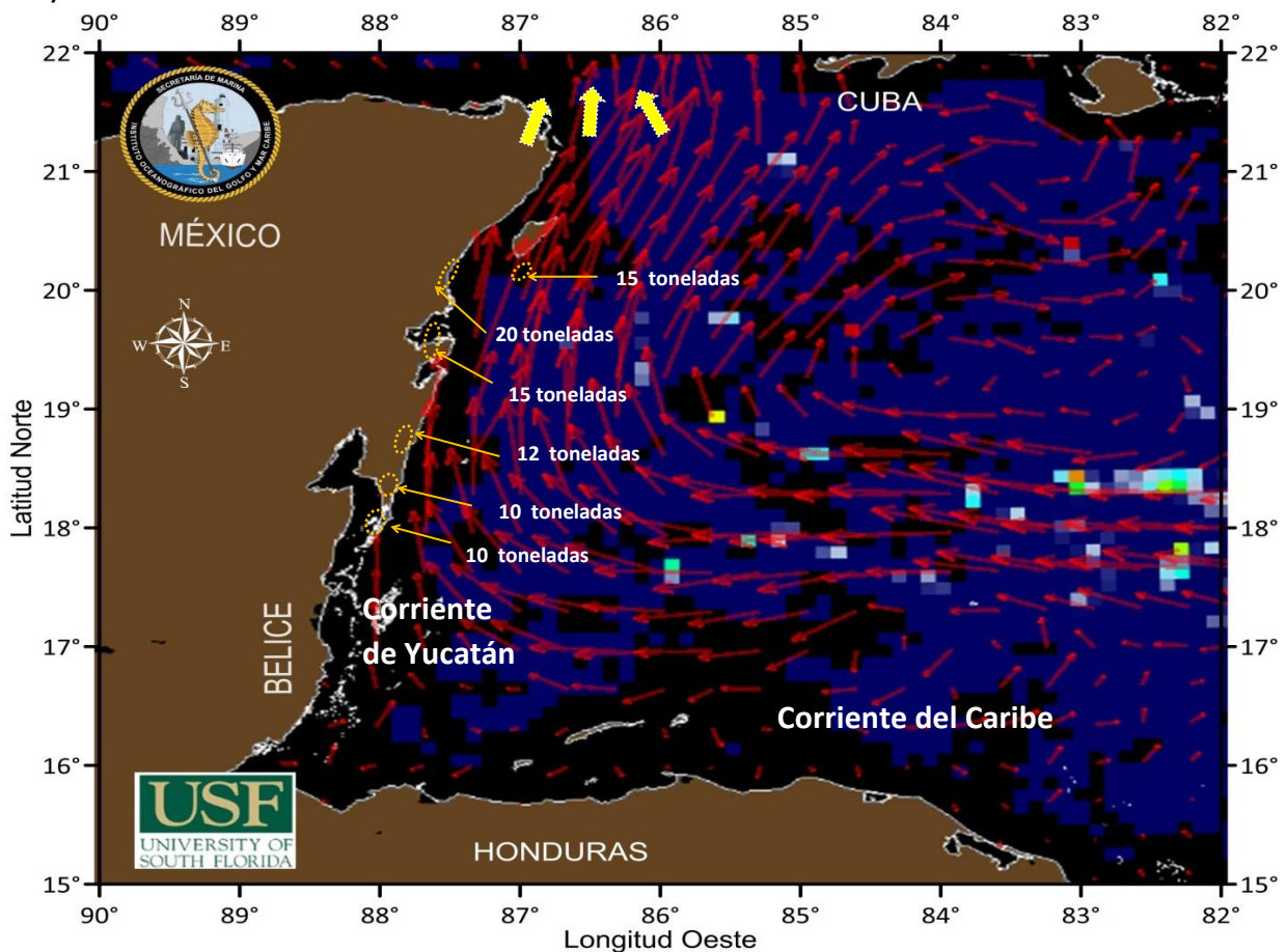
Figura 1.- Cobertura algal (24 de agosto) y la modelación de corrientes superficiales (25 de agosto), obtenidos a partir de datos de la USF.
