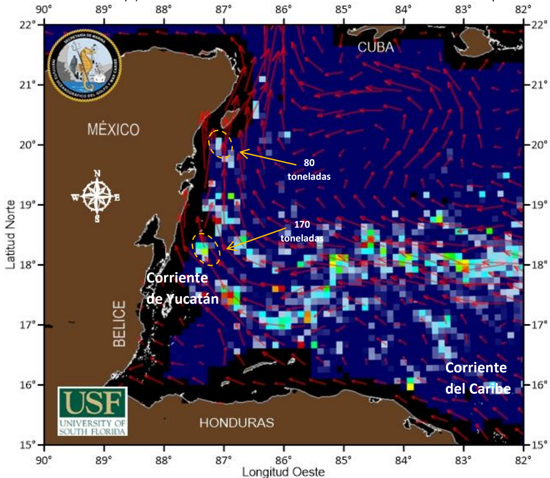
Figura 1.- Cobertura algal (10 de febrero) y modelación de corrientes superficiales (11 de febrero).
