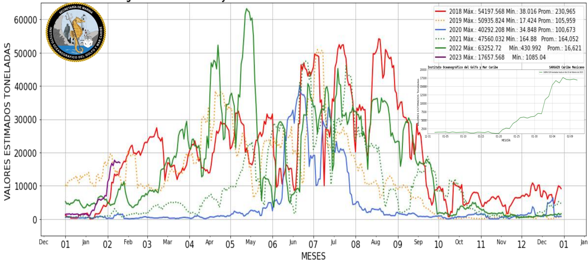
Figura 2.- Valores estimados de la cantidad de sargazo en el Caribe Mexicano. Gráfico comparativo de los años 2018, 2019, 2022 y 2023 (gráfico mayor) y valores estimados del 01 de enero al 10 de febrero del presente año (gráfico superior derecha) obtenidos a partir de datos de la USF.
