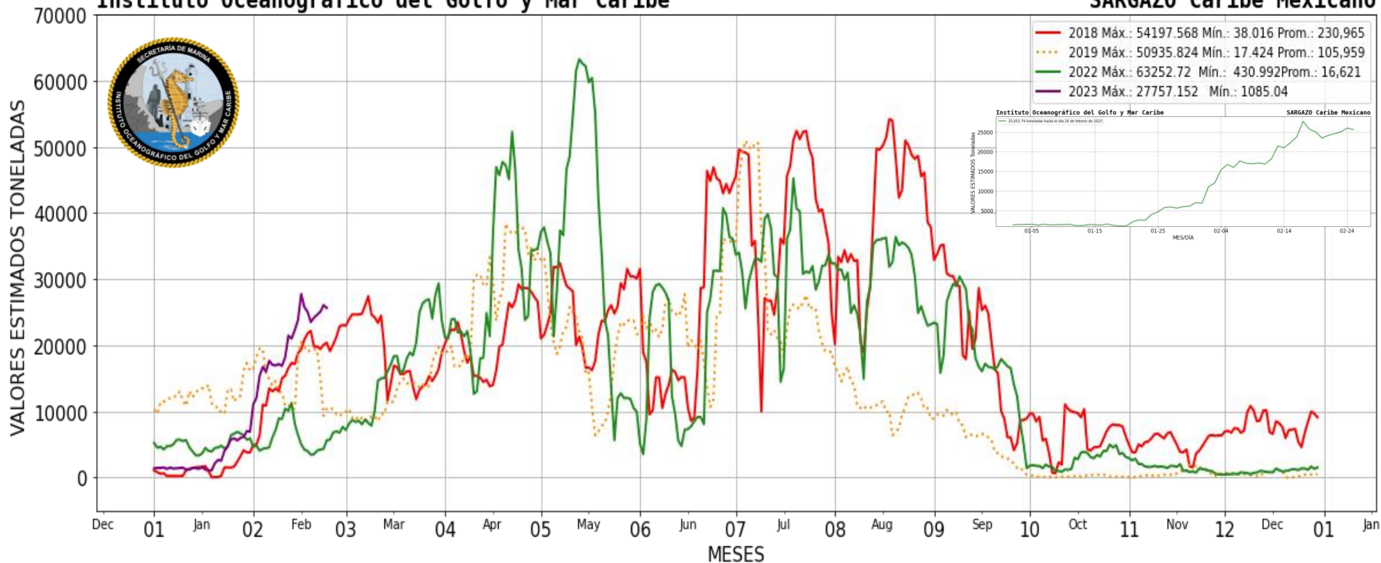
Figura 2.- Valores estimados de la cantidad de sargazo en el Caribe Mexicano. Gráfico comparativo de los años 2018, 2019, 2022 y 2023 (gráfico mayor) y valores estimados del 01 de enero al 24 de febrero del presente año (gráfico superior derecha) obtenidos a partir de datos de la USF.
