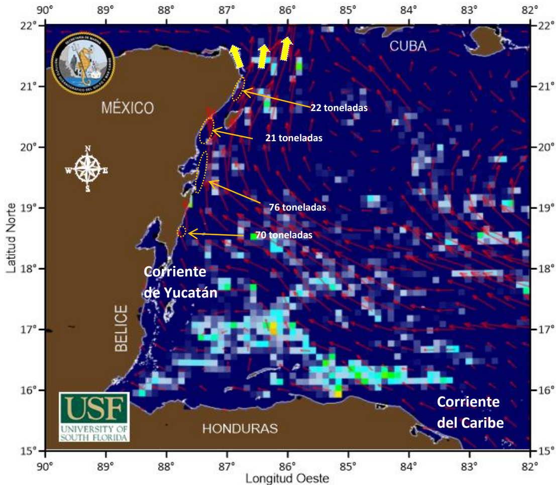
Figura 1.- Cobertura algal (24 de febrero) y modelación de corrientes superficiales (25 de febrero).
