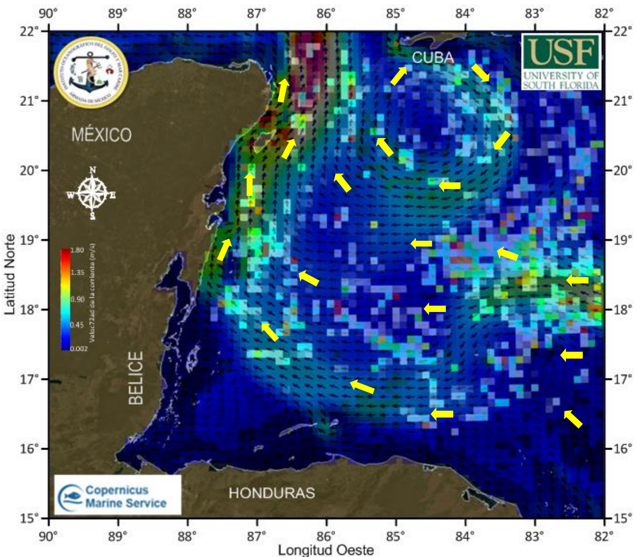
Figura 1.- Cobertura algal (24 de julio) y modelación de corrientes superficiales (25 de julio).
