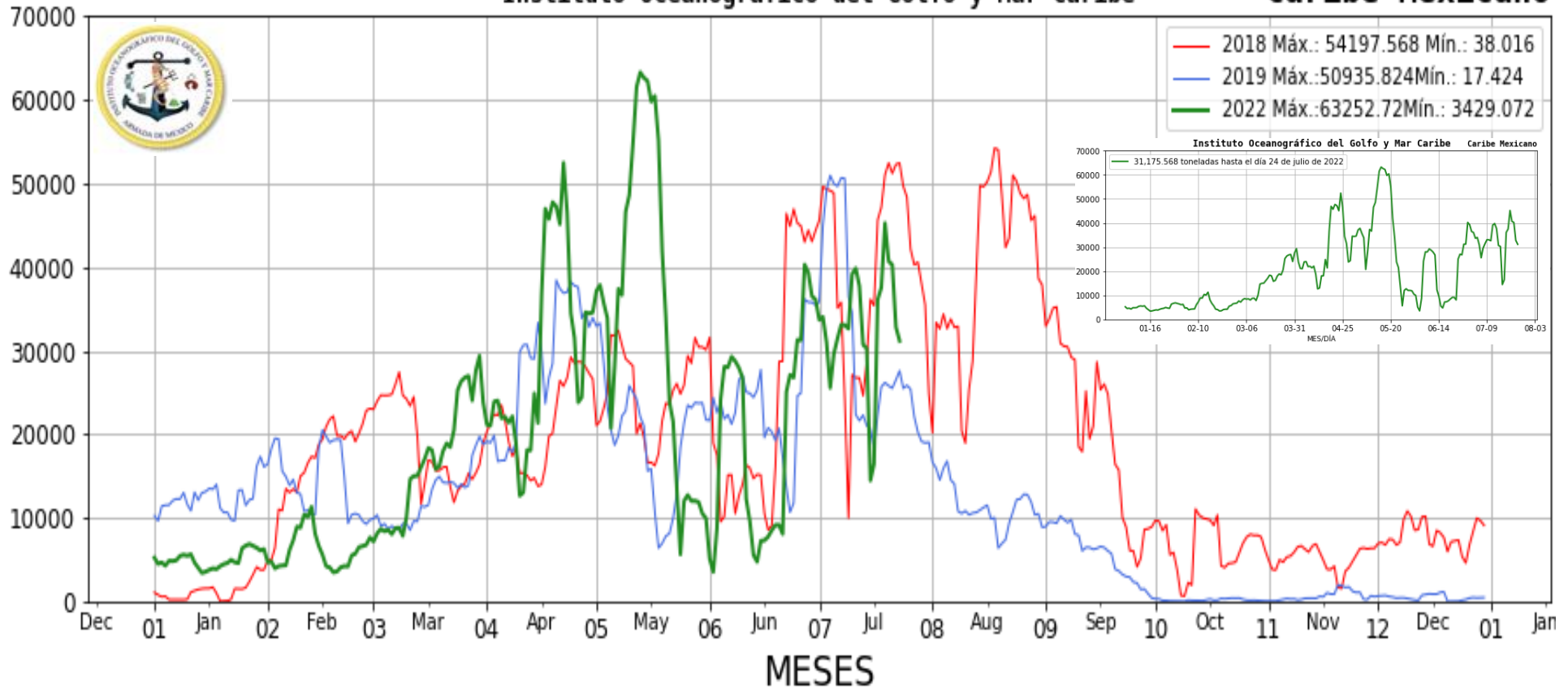
Figura 2.- Valores estimados de la cantidad de sargazo en el Caribe Mexicano. Gráfico comparativo de los años 2018, 2019 y 2022 (gráfico mayor) y valores estimados del 1 de enero al 24 de julio del presente año (gráfico superior derecha) obtenidos a partir de datos de la USF.
