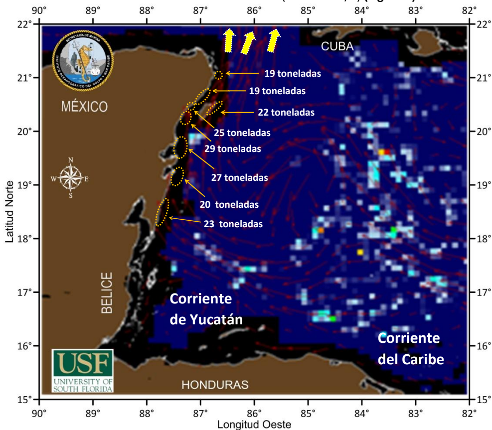
Figura 1.- Cobertura algal (01 de julio) y la modelación de corrientes superficiales (02 de julio), obtenidos a partir de datos de la USF.
