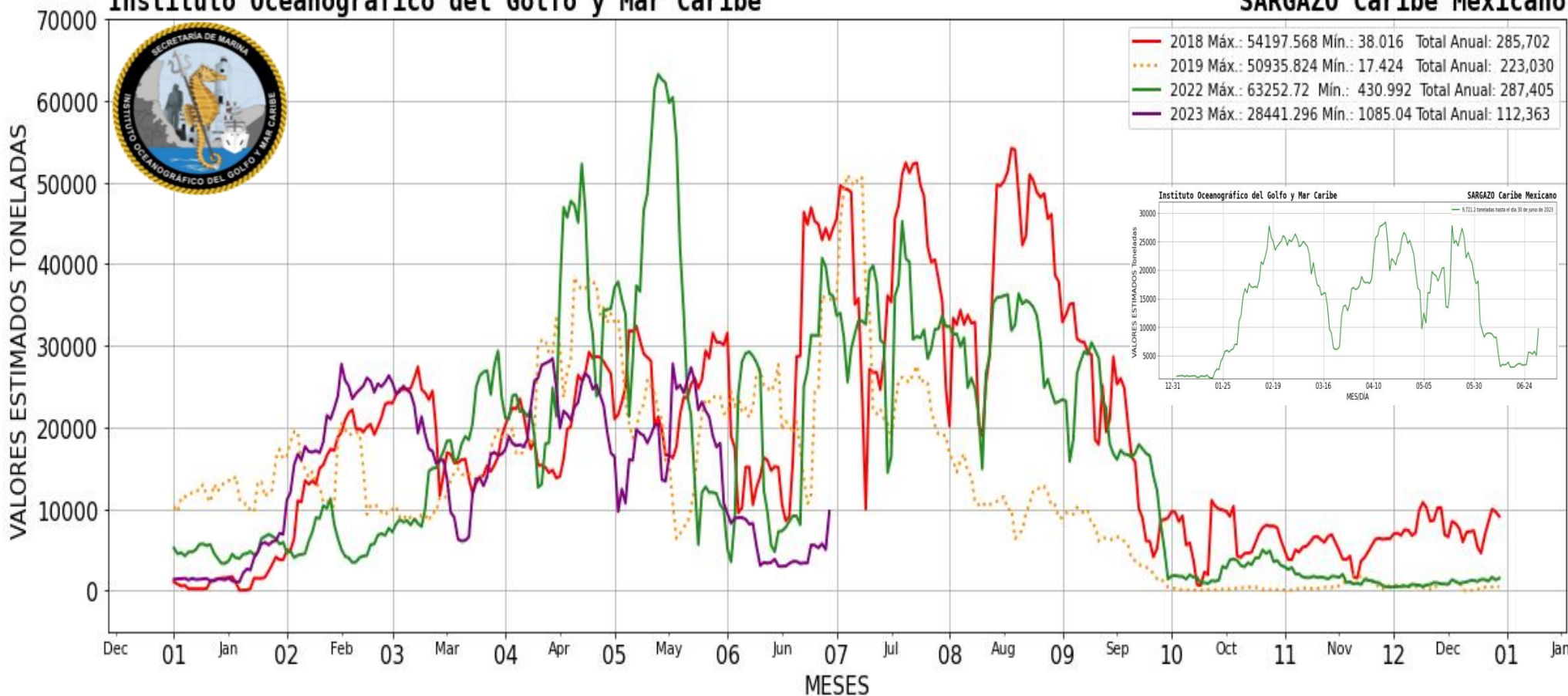
Figura 2.- Presencia aproximada de sargazo en el Caribe Mexicano. Gráfico comparativo de los años 2018, 2019, 2022 y 2023 (gráfico mayor) y valores estimados del 01 de enero al 01 de julio del presente año (gráfico superior derecho) obtenidos a partir de datos de la USF.
