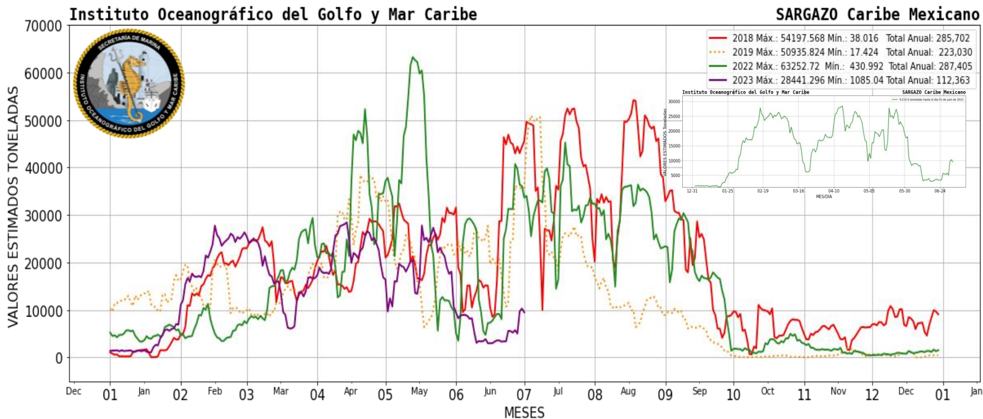
Figura 2.- Presencia aproximada de sargazo en el Caribe Mexicano. Gráfico comparativo de los años 2018, 2019, 2022 y 2023 (gráfico mayor) y valores estimados del 01 de enero al 02 de julio del presente año (gráfico superior derecho) obtenidos a partir de datos de la USF.
