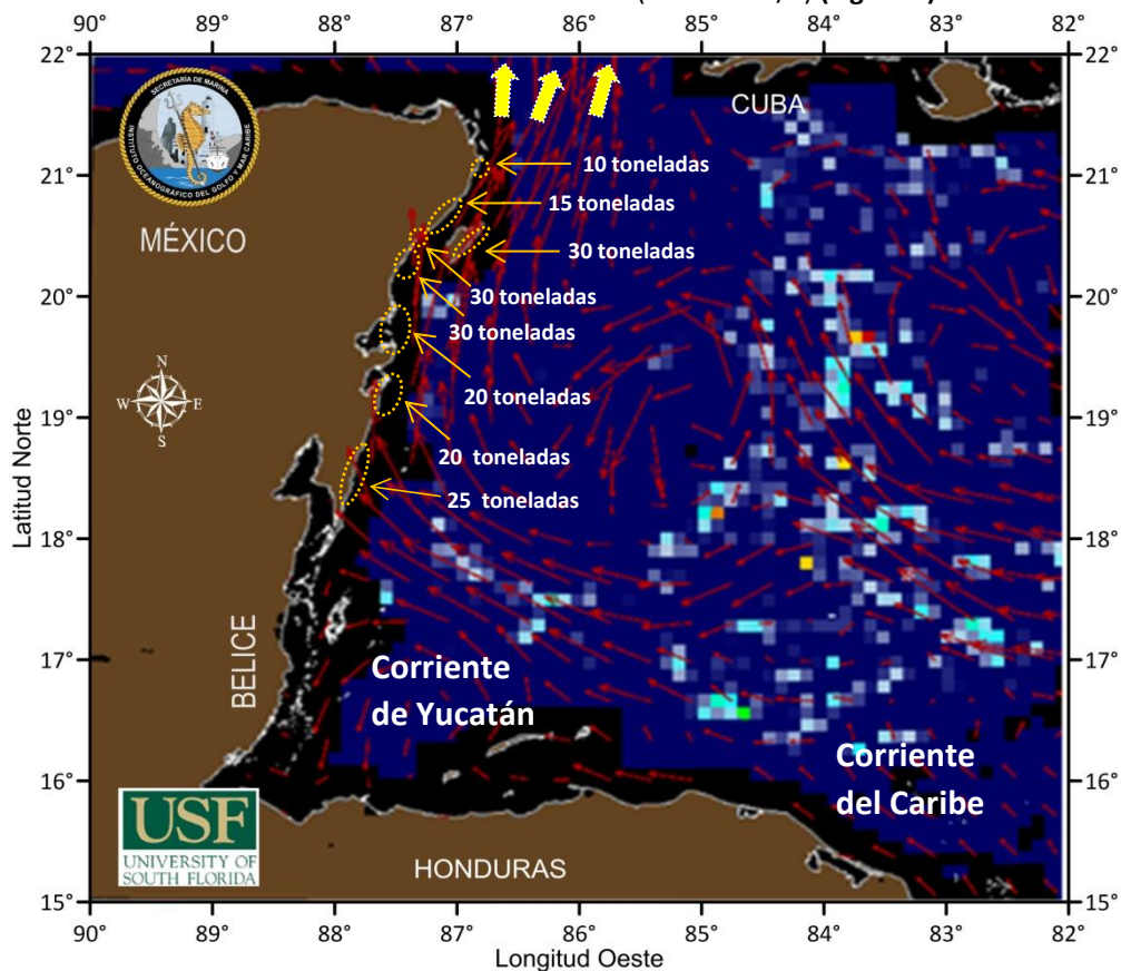
Figura 1.- Cobertura algal (02 de julio) y la modelación de corrientes superficiales (03 de julio), obtenidos a partir de datos de la USF.
