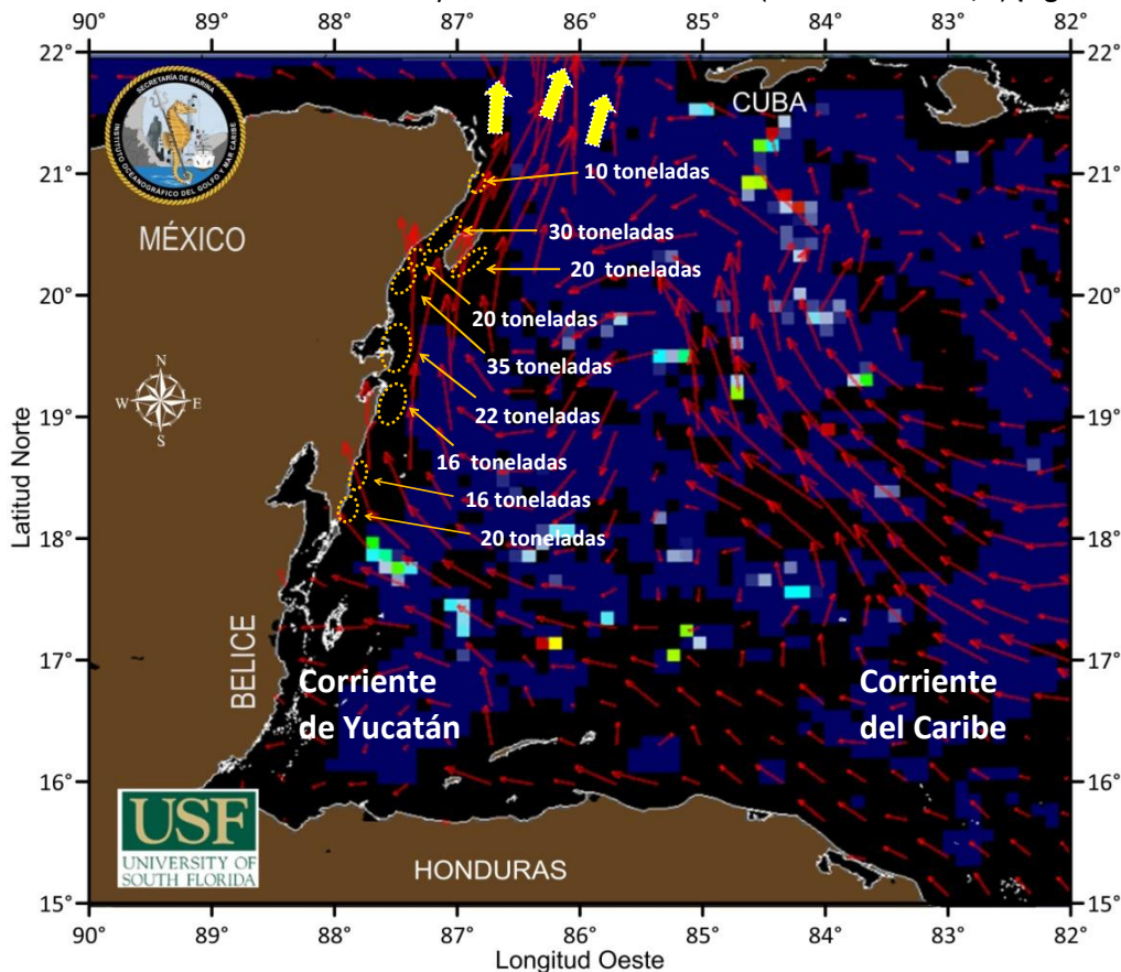
Figura 1.- Cobertura algal (09 de julio) y la modelación de corrientes superficiales (10 de julio), obtenidos a partir de datos de la USF.
