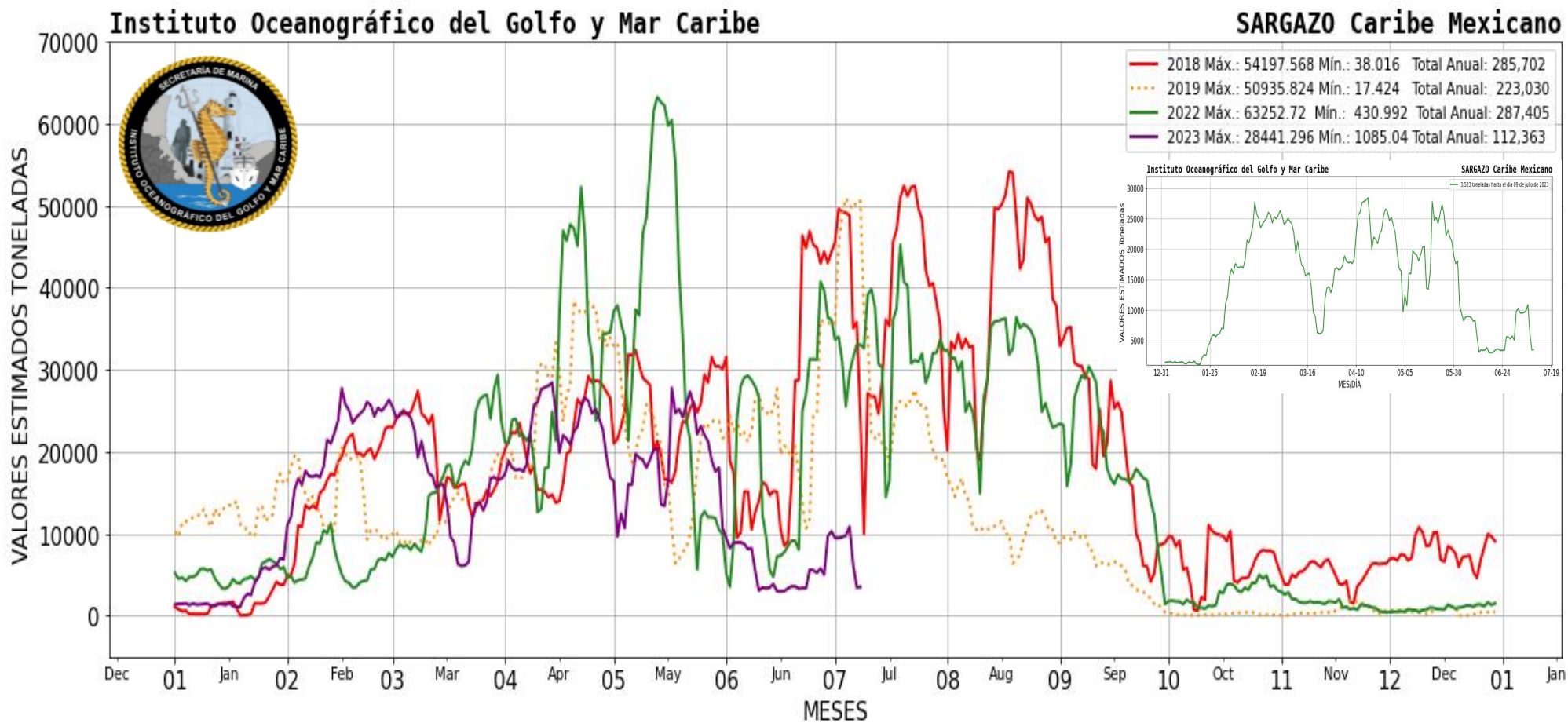
Figura 2.- Presencia aproximada de sargazo en el Caribe Mexicano. Gráfico comparativo de los años 2018, 2019, 2022 y 2023 (gráfico mayor) y valores estimados del 01 de enero al 09 de julio del presente año (gráfico superior derecho) obtenidos a partir de datos de la USF.
