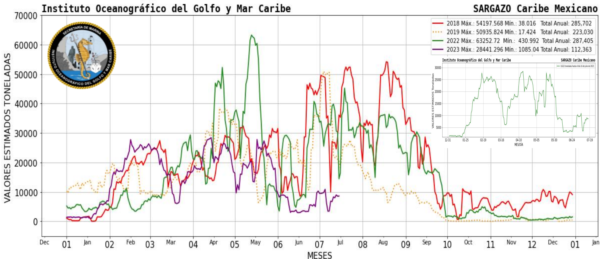
Figura 2.- Presencia aproximada de sargazo en el Caribe Mexicano. Gráfico comparativo de los años 2018, 2019, 2022 y 2023 (gráfico mayor) y valores estimados del 01 de enero al 16 de julio del presente año (gráfico superior derecho) obtenidos a partir de datos de la USF.
