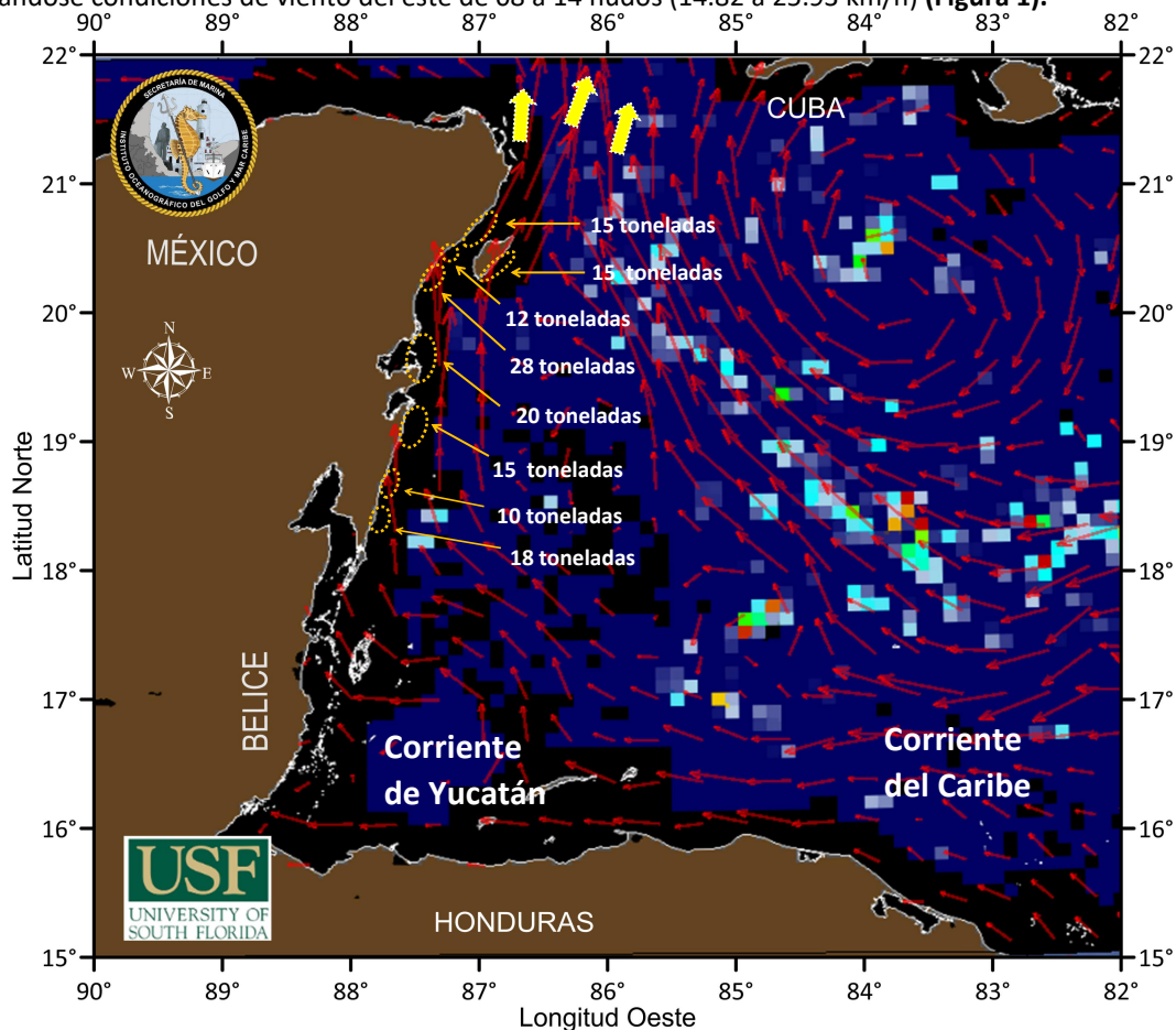
Figura 1.- Cobertura algal (16 de julio) y la modelación de corrientes superficiales (17 de julio), obtenidos a partir de datos de la USF.
