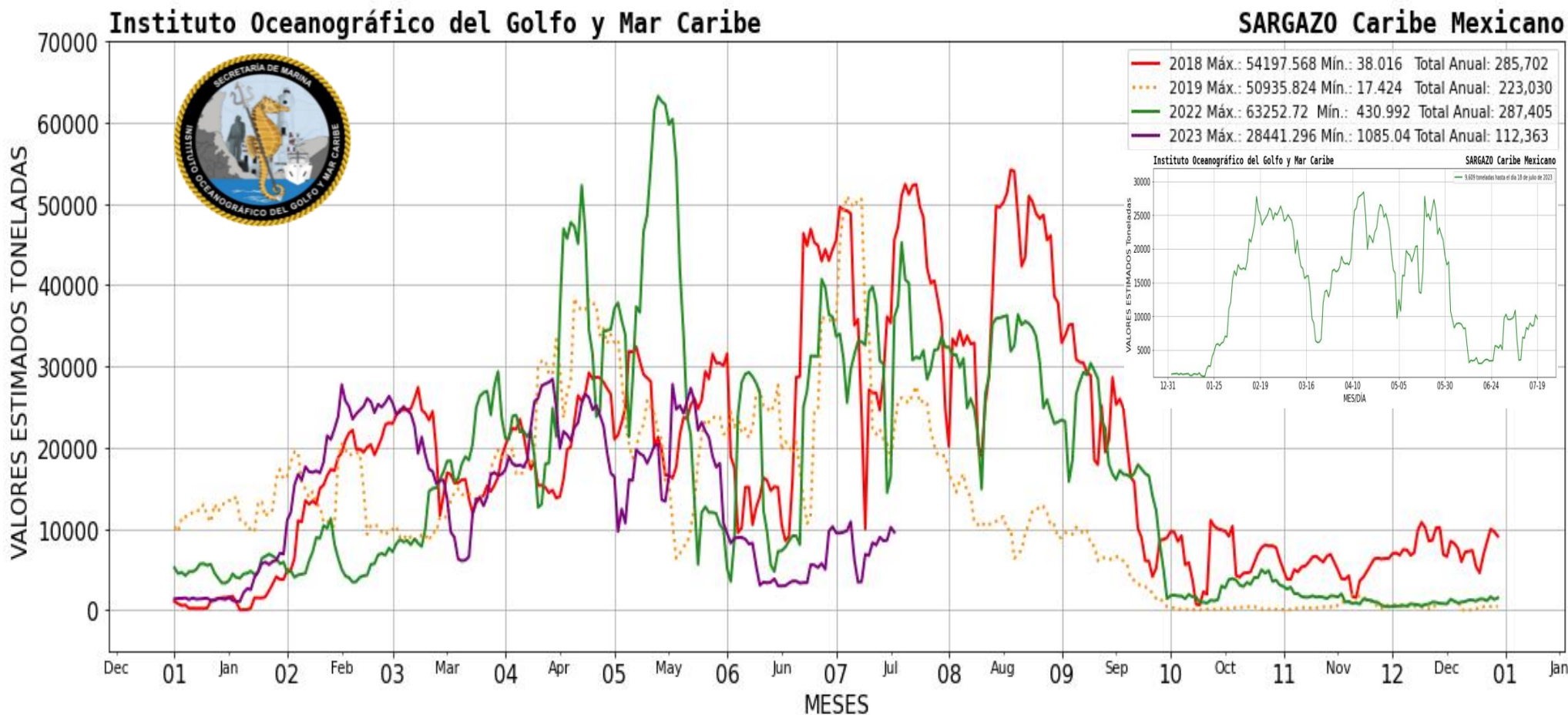
Figura 2.- Presencia aproximada de sargazo en el Caribe Mexicano. Gráfico comparativo de los años 2018, 2019, 2022 y 2023 (gráfico mayor) y valores estimados del 01 de enero al 18 de julio del presente año (gráfico superior derecho) obtenidos a partir de datos de la USF.
