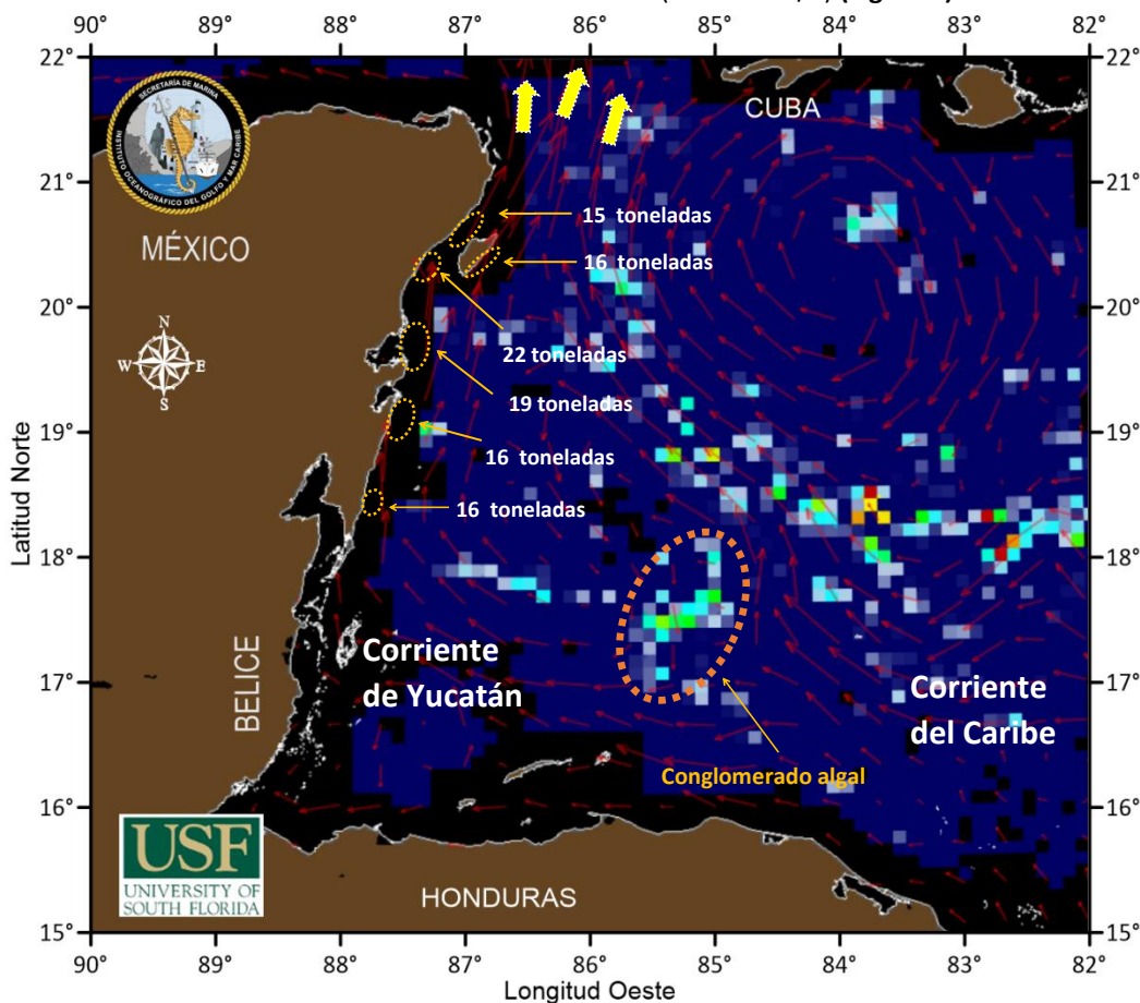
Figura 1.- Cobertura algal (18 de julio) y la modelación de corrientes superficiales (19 de julio), obtenidos a partir de datos de la USF.
