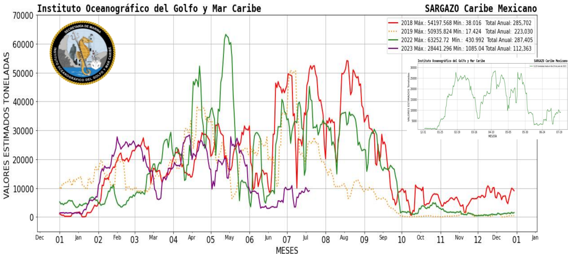
Figura 2.- Presencia aproximada de sargazo en el Caribe Mexicano. Gráfico comparativo de los años 2018, 2019, 2022 y 2023 (gráfico mayor) y valores estimados del 01 de enero al 20 de julio del presente año (gráfico superior derecho) obtenidos a partir de datos de la USF.
