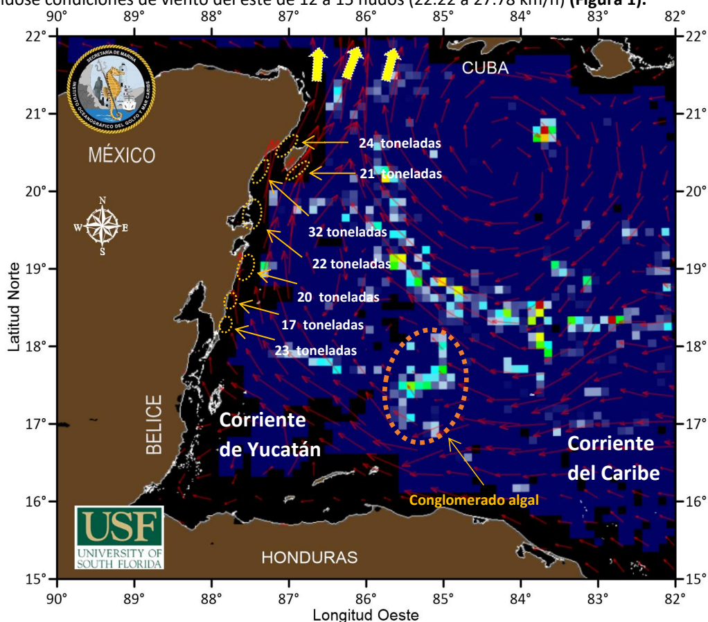
Figura 1.- Cobertura algal (20 de julio) y la modelación de corrientes superficiales (21 de julio), obtenidos a partir de datos de la USF.
