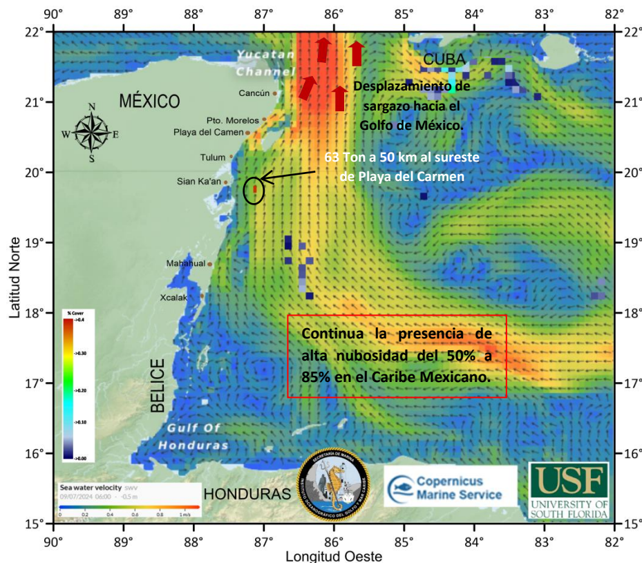
Figura 2.- Cobertura algal (08 de julio) y la modelación de corrientes superficiales (09 de julio), obtenidos a partir de datos de la USF.
