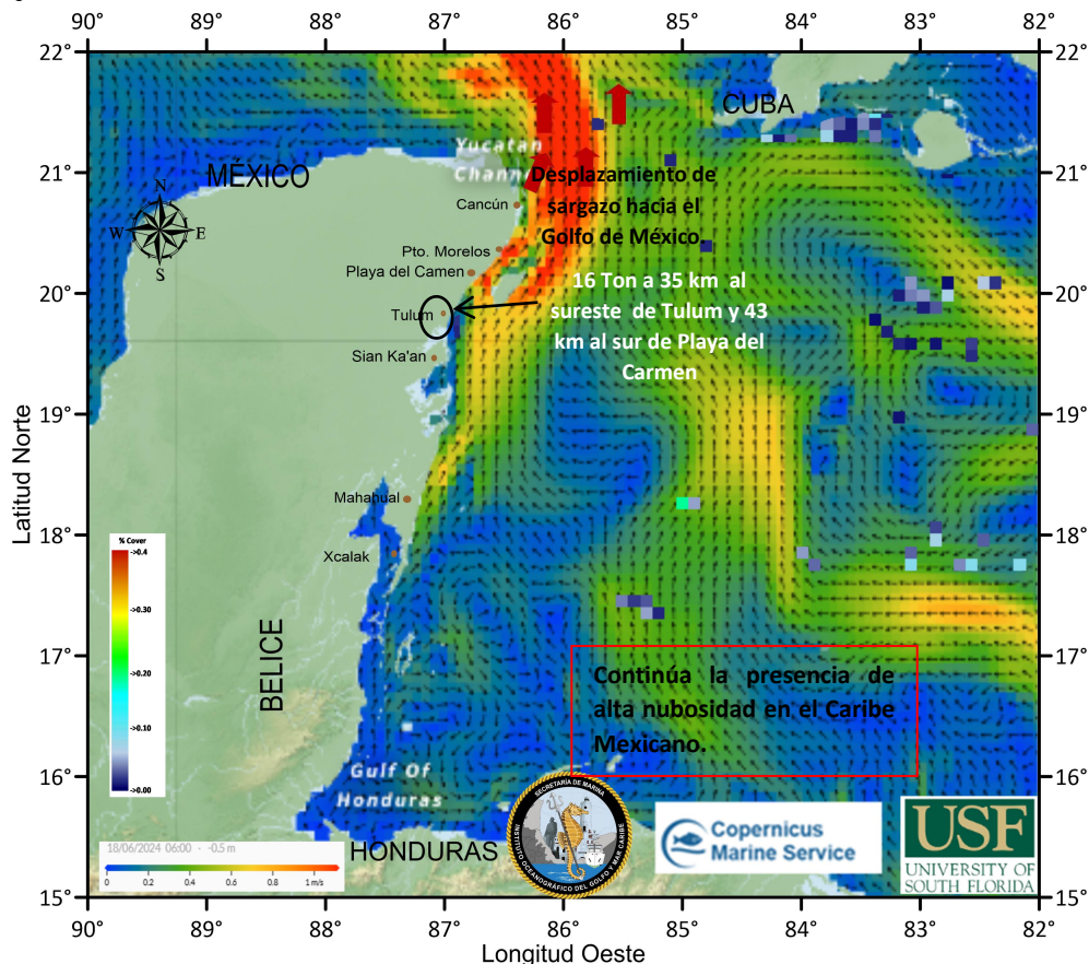
Figura 2.- Cobertura algal ( 17 de julio ) y la modelación de corrientes superficiales ( 18 de julio ), obtenidos a partir de datos de la USF.
