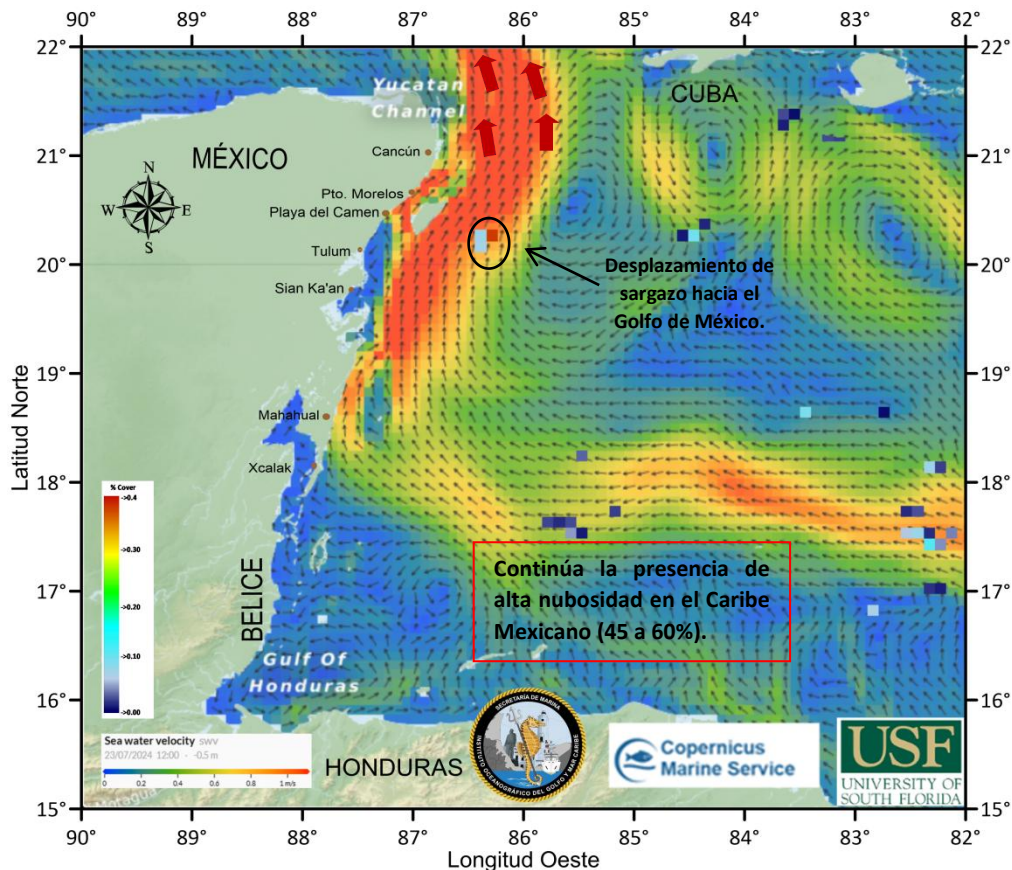
Figura 2.- Cobertura algal (22 de julio) y la modelación de corrientes superficiales (23 de julio), obtenidos a partir de datos de la USF.
