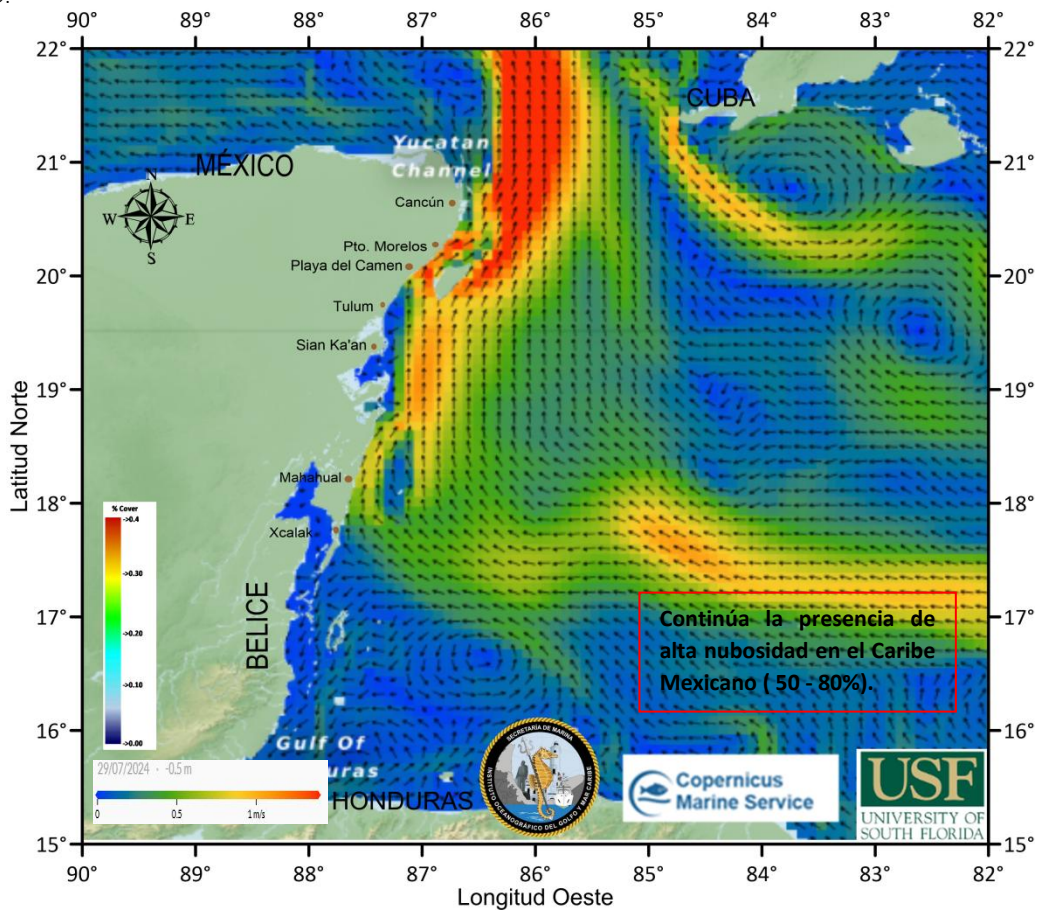
Figura 2.- Cobertura algal ( 28 de julio ) y la modelación de corrientes superficiales ( 29 de julio ), obtenidos a partir de datos de la USF.
