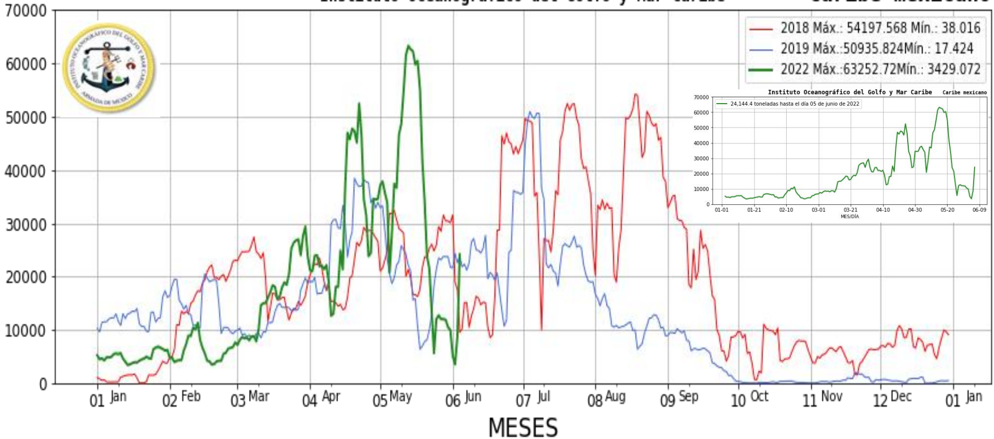
Figura 2.- Valores estimados de la cantidad de sargazo en el Caribe Mexicano. Gráfico comparativo de los años 2018, 2019 y 2022 (gráfico mayor) y valores estimados del 01 de enero al 05 de junio del presente año (gráfico superior derecha) obtenidos a partir de datos de la USF.
