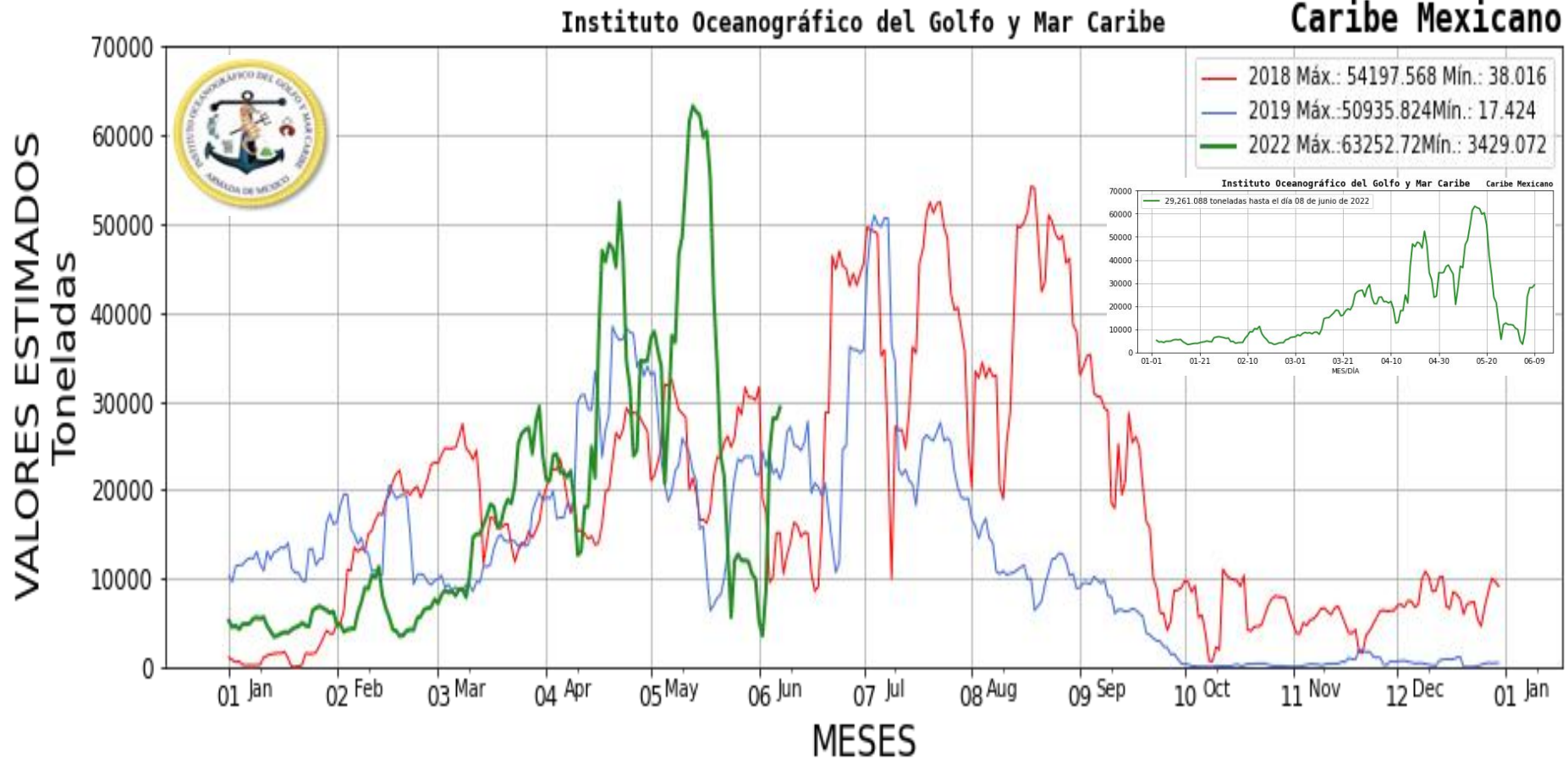
Figura 2.- Valores estimados de la cantidad de sargazo en el Caribe Mexicano. Gráfico comparativo de los años 2018, 2019 y 2022 (gráfico mayor) y valores estimados del 01 de enero al 08 de junio del presente año (gráfico superior derecha) obtenidos a partir de datos de la USF.
