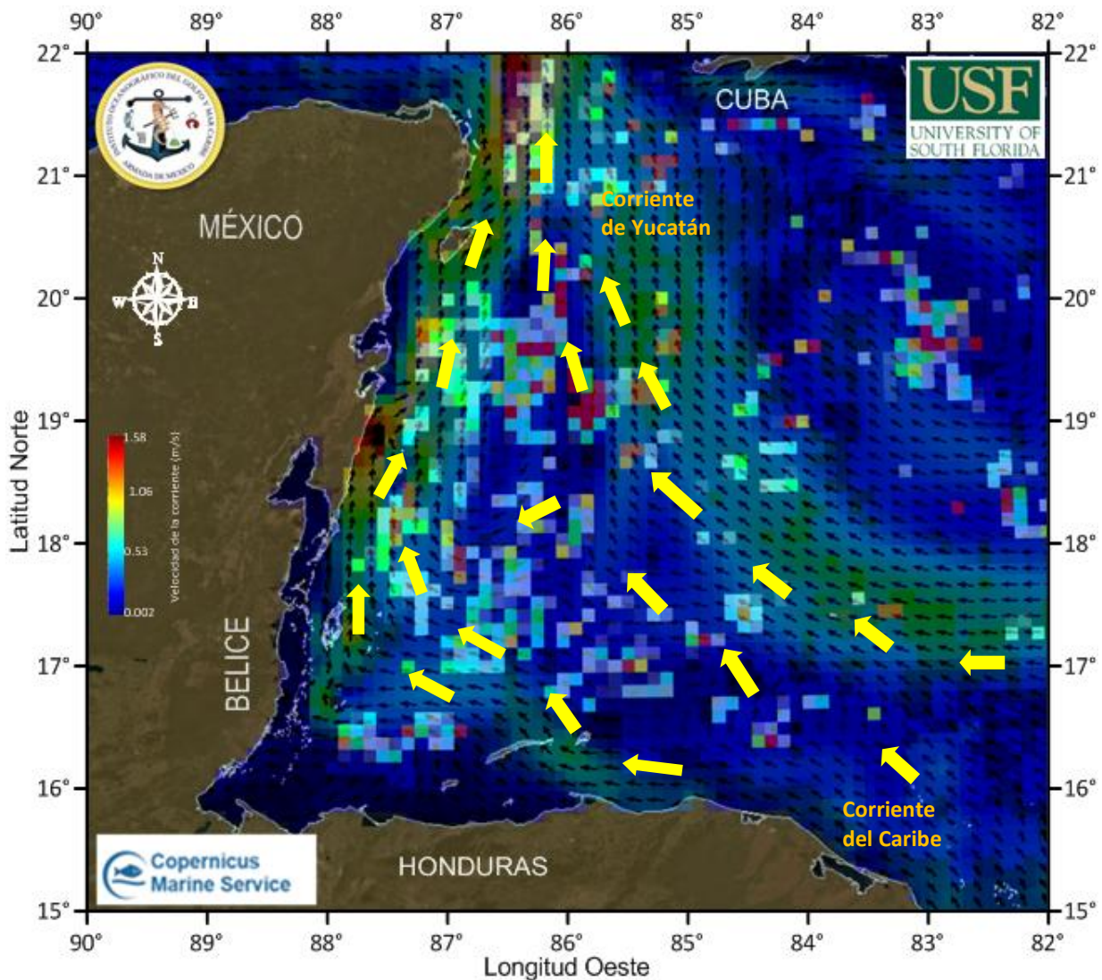
Figura 1.- Cobertura algal (08 de junio) y modelación de corrientes superficiales (09 de junio).
