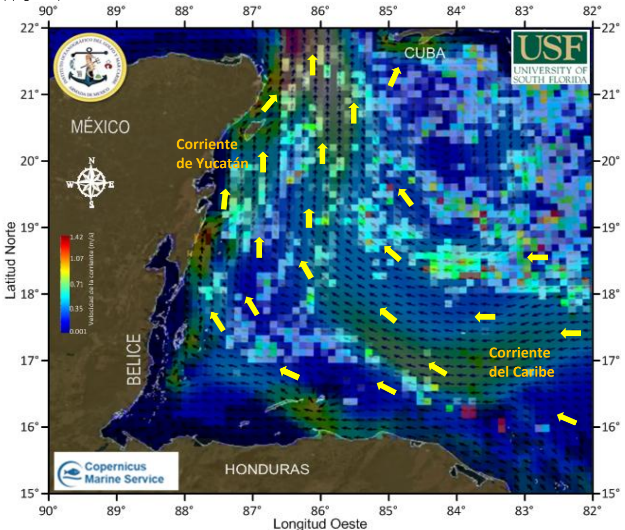
Figura 1.- Cobertura algal (28 de junio) y modelación de corrientes superficiales (29 de junio).
