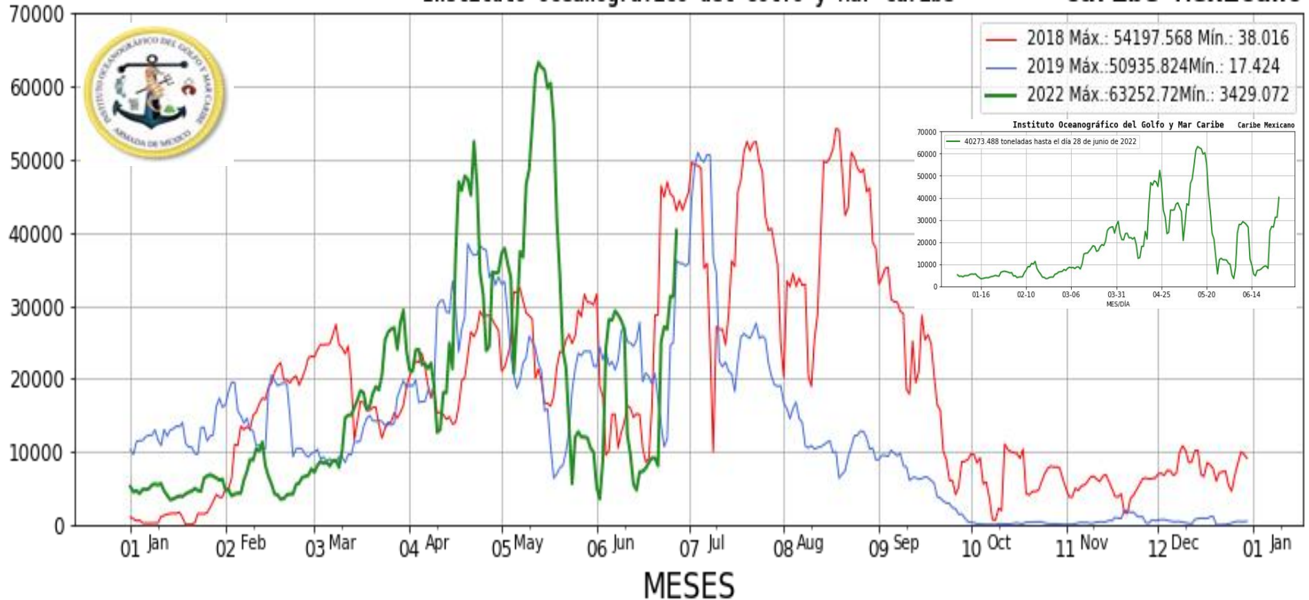
Figura 2.- Valores estimados de la cantidad de sargazo en el Caribe Mexicano. Gráfico comparativo de los años 2018, 2019 y 2022 (gráfico mayor) y valores estimados del 01 de enero al 28 de junio del presente año (gráfico superior derecha) obtenidos a partir de datos de la USF.
