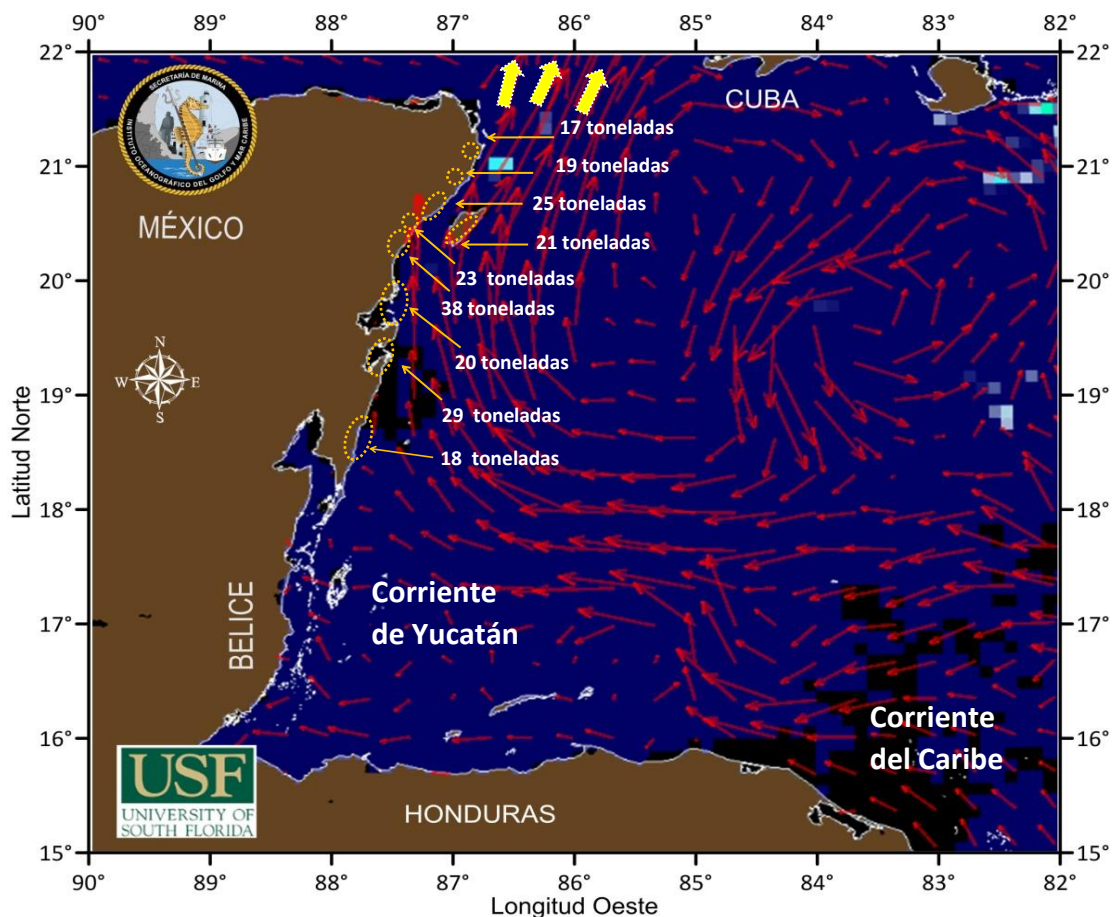
Figura 1.- Cobertura algal (20 de junio) y la modelación de corrientes superficiales (21 de junio), obtenidos a partir de datos de la USF.
