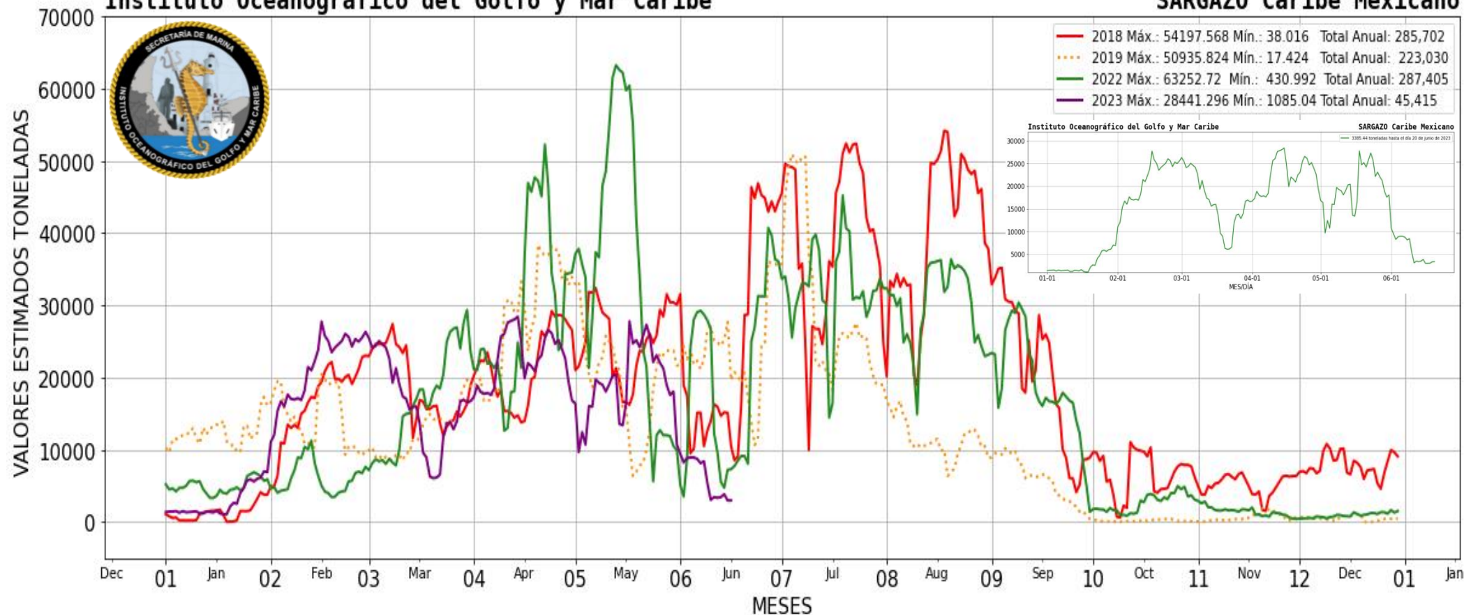
Figura 2.- Presencia aproximada de sargazo en el Caribe Mexicano. Gráfico comparativo de los años 2018, 2019, 2022 y 2023 (gráfico mayor) y valores estimados del 01 de enero al 20 de junio del presente año (gráfico superior derecha) obtenidos a partir de datos de la USF.
