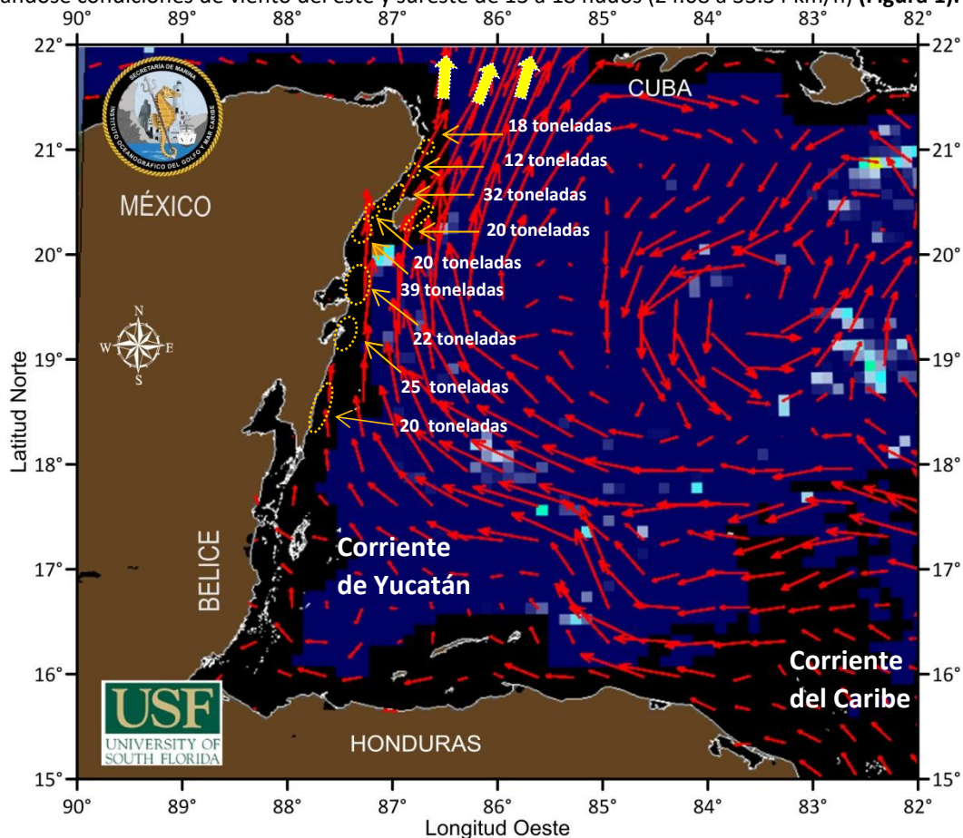
Figura 1.- Cobertura algal (21 de junio) y la modelación de corrientes superficiales (22 de junio), obtenidos a partir de datos de la USF.
