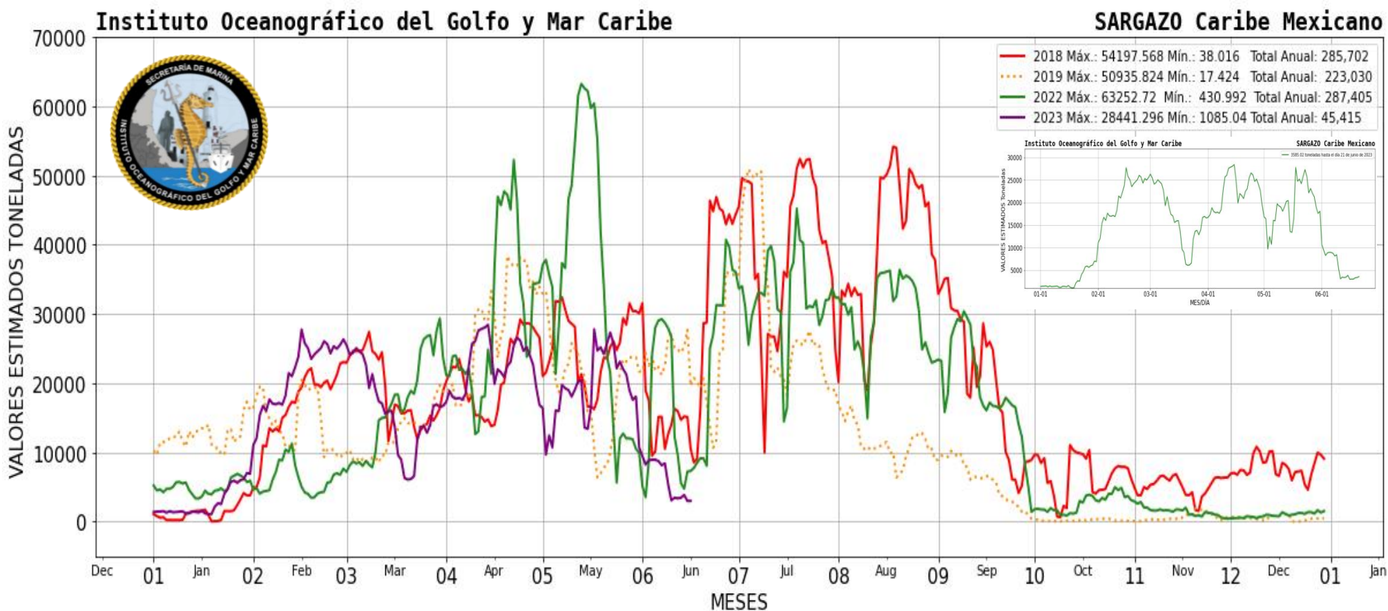
Figura 2.- Presencia aproximada de sargazo en el Caribe Mexicano. Gráfico comparativo de los años 2018, 2019, 2022 y 2023 (gráfico mayor) y valores estimados del 01 de enero al 21 de junio del presente año (gráfico superior derecha) obtenidos a partir de datos de la USF.
