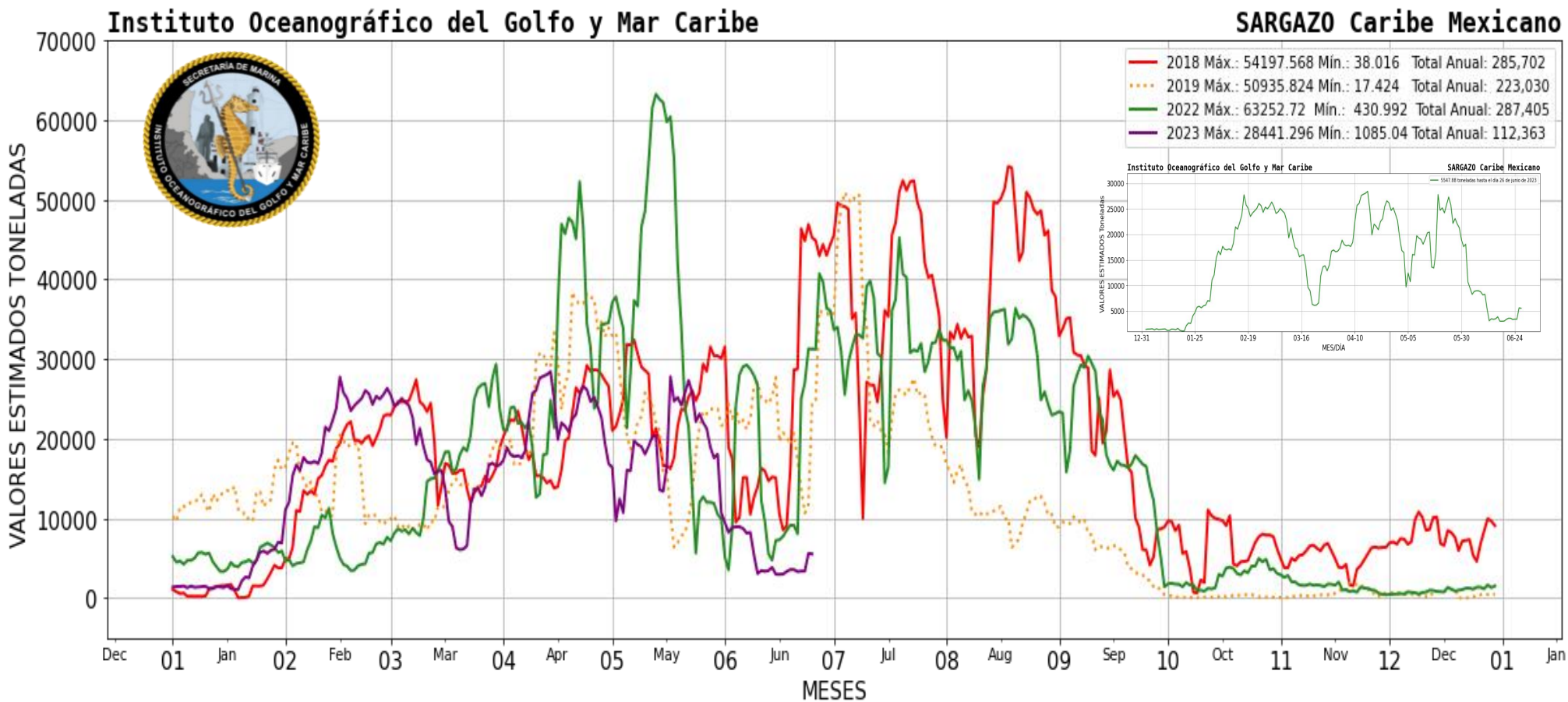
Figura 2.- Presencia aproximada de sargazo en el Caribe Mexicano. Gráfico comparativo de los años 2018, 2019, 2022 y 2023 (gráfico mayor) y valores estimados del 01 de enero al 26 de junio del presente año (gráfico superior derecho) obtenidos a partir de datos de la USF.
