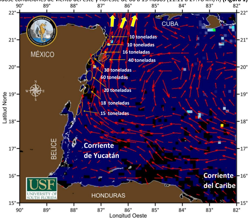
Figura 1.- Cobertura algal (26 de junio) y la modelación de corrientes superficiales (27 de junio), obtenidos a partir de datos de la USF.
