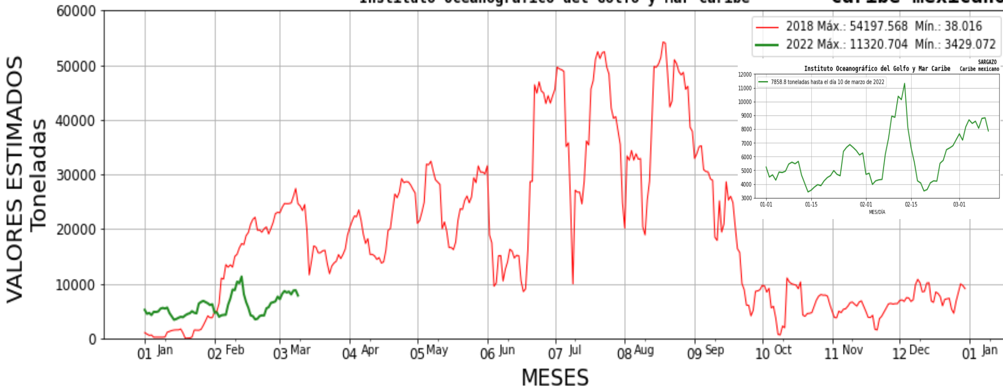
Figura 2.- Valores estimados de la cantidad de sargazo en el Caribe Mexicano. Gráfico comparativo de los años 2018 y 2022 (gráfico mayor) y Valores estimados del 01 de enero al 10 de marzo del presente año (gráfico menor, situado en la parte superior derecha) obtenidos a partir de datos de la USF.
