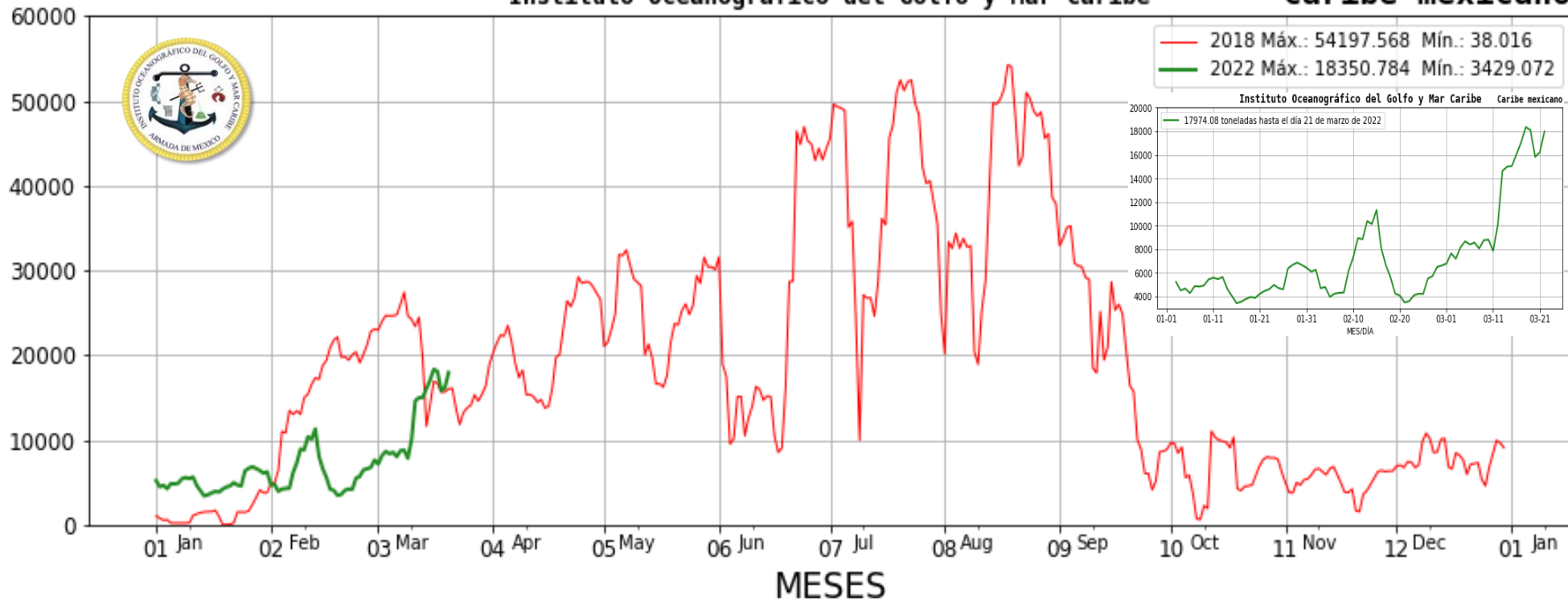
Figura 2.- Valores estimados de la cantidad de sargazo en el Caribe Mexicano. Gráfico comparativo de los años 2018 y 2022 (gráfico mayor) y Valores estimados del 01 de enero al 21 de marzo del presente año (gráfico menor, situado en la parte superior derecha) obtenidos a partir de datos de la USF.
