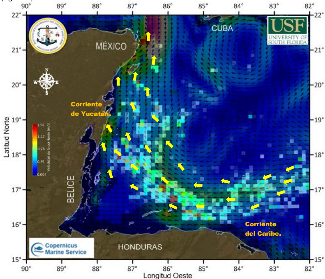
Figura 1.- Cobertura algal (21 de marzo) y modelación de corrientes superficiales (22 de marzo).
