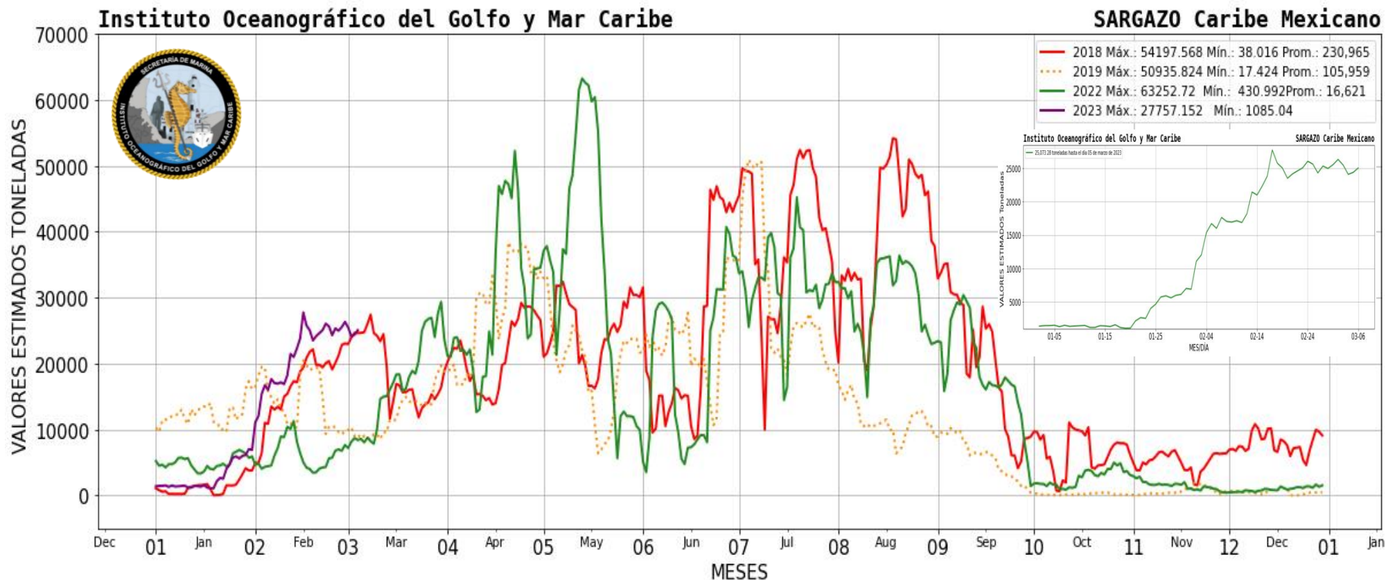
Figura 2.- Valores estimados de la cantidad de sargazo en el Caribe Mexicano. Gráfico comparativo de los años 2018, 2019, 2022 y 2023 (gráfico mayor) y valores estimados del 01 de enero al 05 de marzo del presente año (gráfico superior derecha) obtenidos a partir de datos de la USF.
