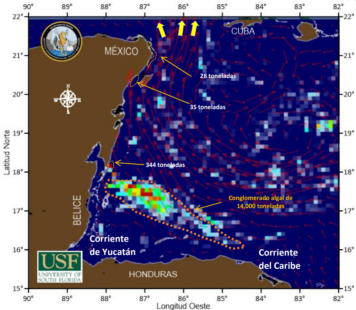
Figura 1.- Cobertura algal (04 de marzo) y modelación de corrientes superficiales (05 de marzo).
