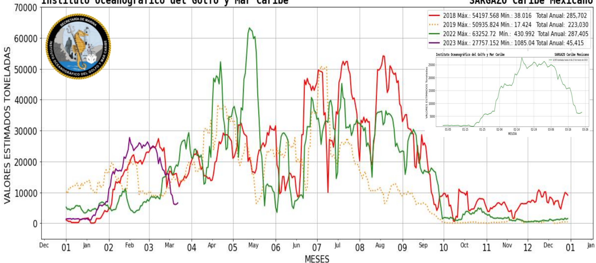
Figura 2.- Valores estimados de la cantidad de sargazo en el Caribe Mexicano. Gráfico comparativo de los años 2018, 2019, 2022 y 2023 (gráfico mayor) y valores estimados del 01 de enero al 23 de marzo del presente año (gráfico superior derecha) obtenidos a partir de datos de la USF.
