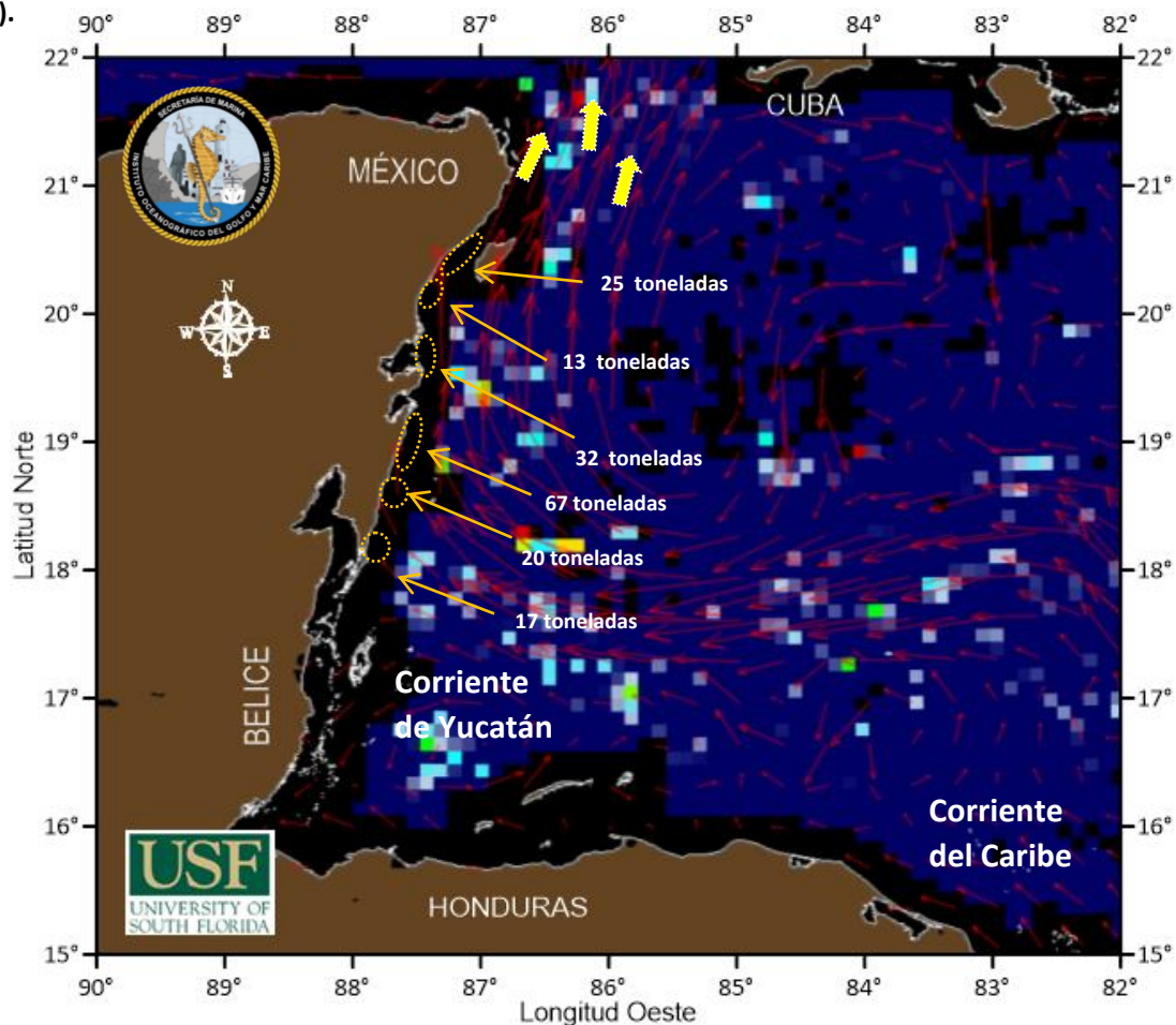
Figura 1.- Cobertura algal (23 de marzo) y modelación de corrientes superficiales (24 de marzo).
