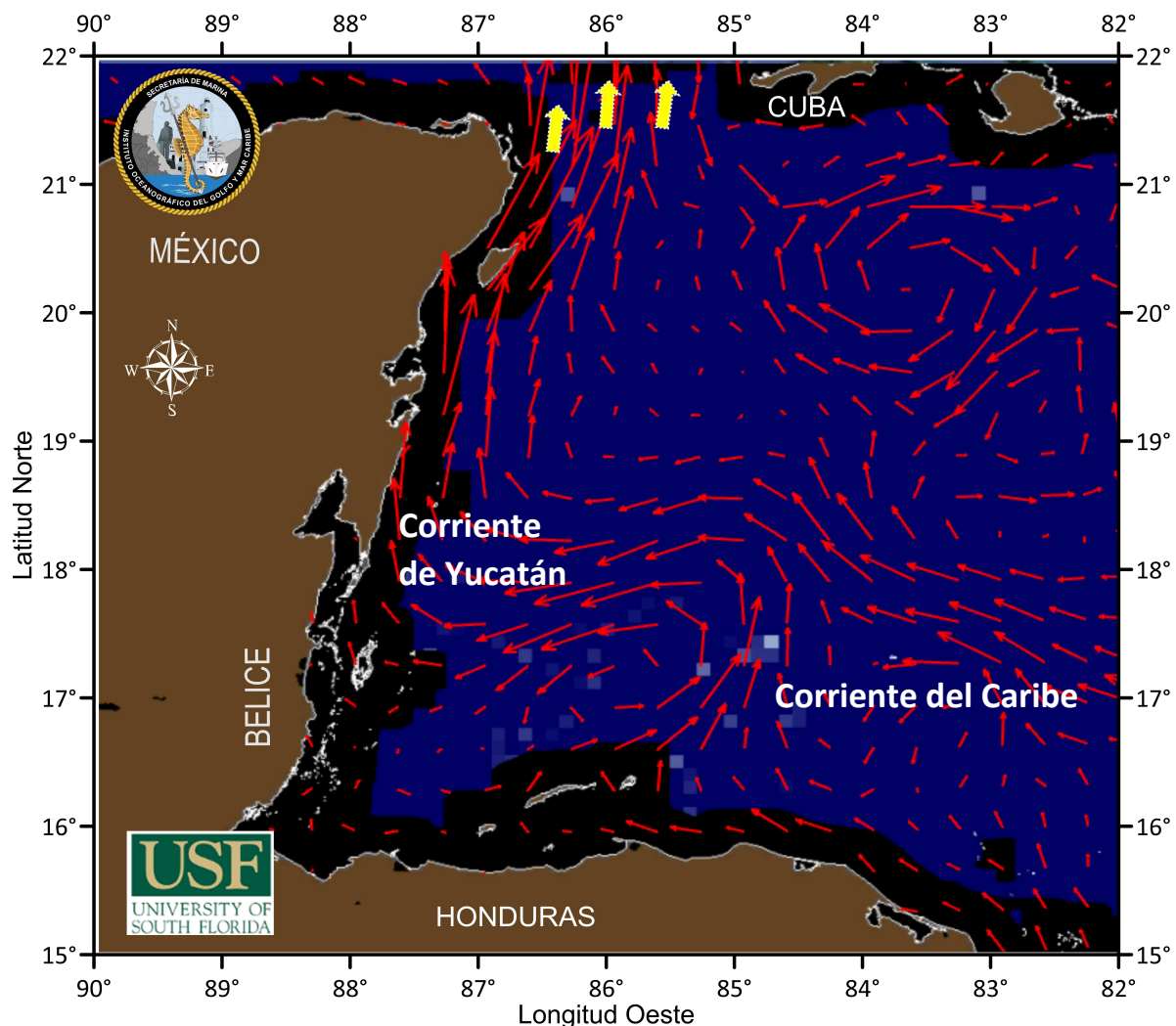
Figura 1.-Cobertura algal (03 de marzo) y la modelación de corrientes superficiales (04 de marzo), obtenidos a partir de datos de la USF.
