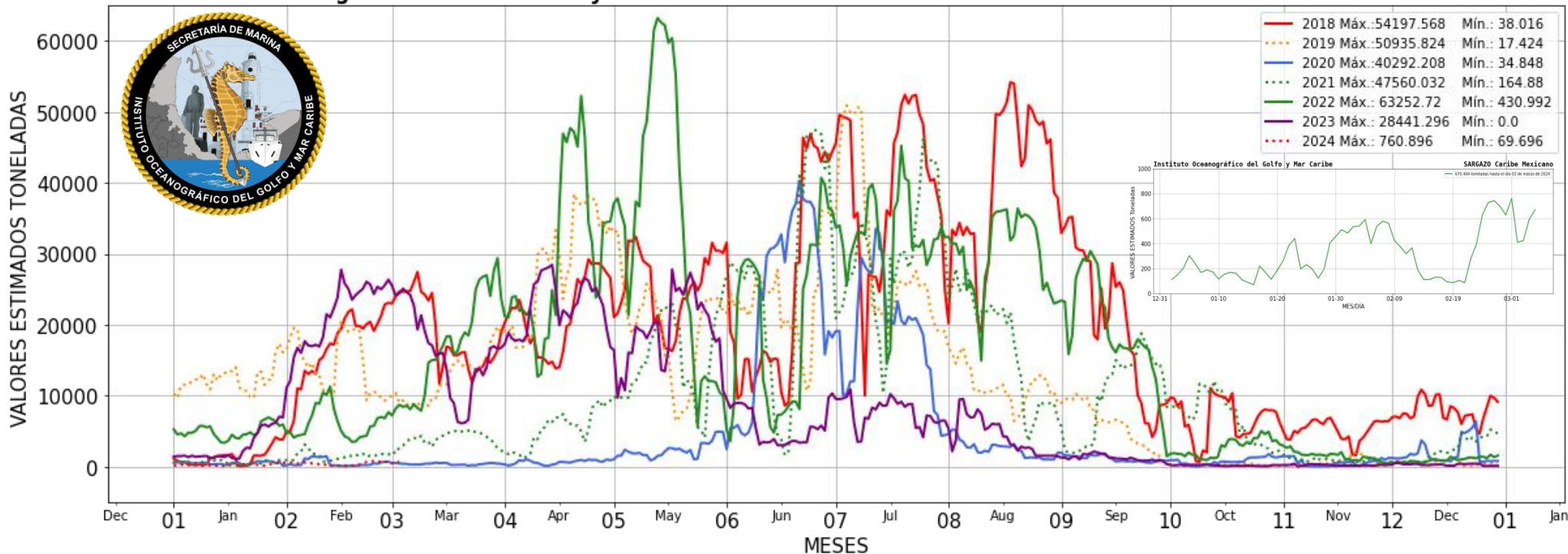
Figura 2.- Presencia aproximada de sargazo en el Caribe Mexicano. Gráfico comparativo de los años 2018-2024 (gráfico mayor) y valores estimados del 01 de enero al 03 de marzo del presente año (gráfico superior derecho) obtenidos a partir de datos de la USF.
