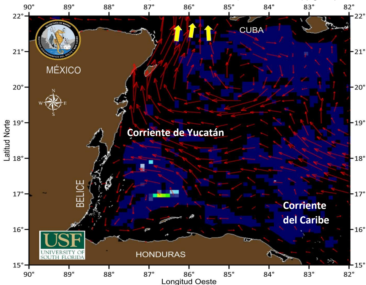
Figura 1.- Cobertura algal (21 de marzo) y la modelación de corrientes superficiales (22 de marzo), obtenidos a partir de datos de la USF.
