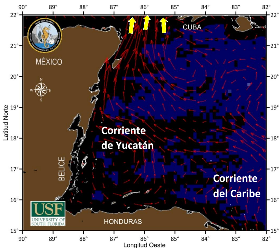
Figura 1.- Cobertura algal (27 de marzo) y la modelación de corrientes superficiales (28 de marzo), obtenidos a partir de datos de la USF.
