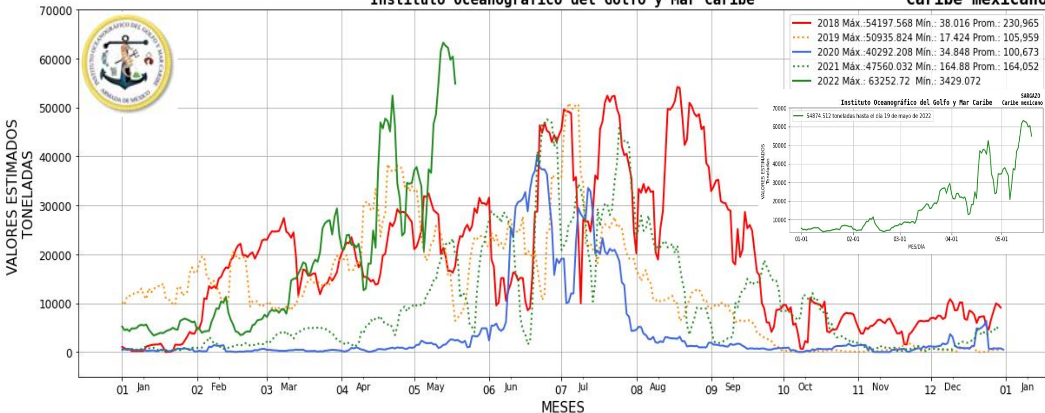
Figura 2.- Valores estimados de la cantidad de sargazo en el Caribe Mexicano. Gráfico comparativo de los años 2018, 2019, 2020, 2021 y 2022 (gráfico mayor) y valores estimados del 01 de enero al 19 de mayo del presente año (gráfico superior derecha) obtenidos a partir de datos de la USF.
