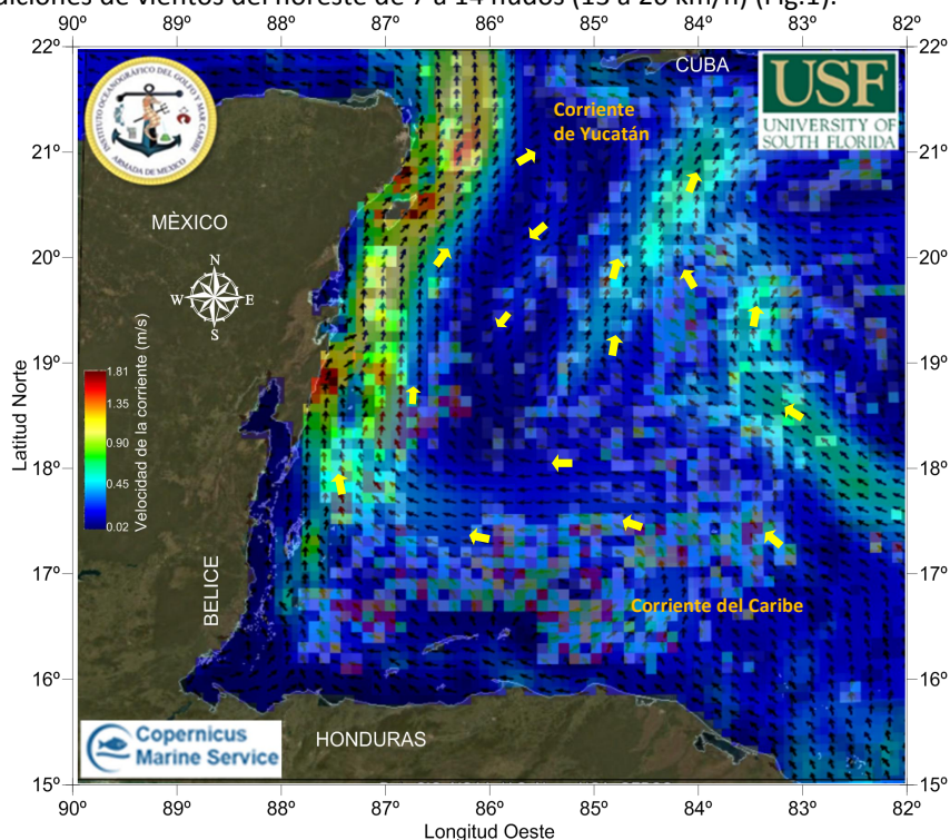
Figura 1.- Cobertura algal (19 de mayo) y modelación de corrientes superficiales (20 de mayo).
