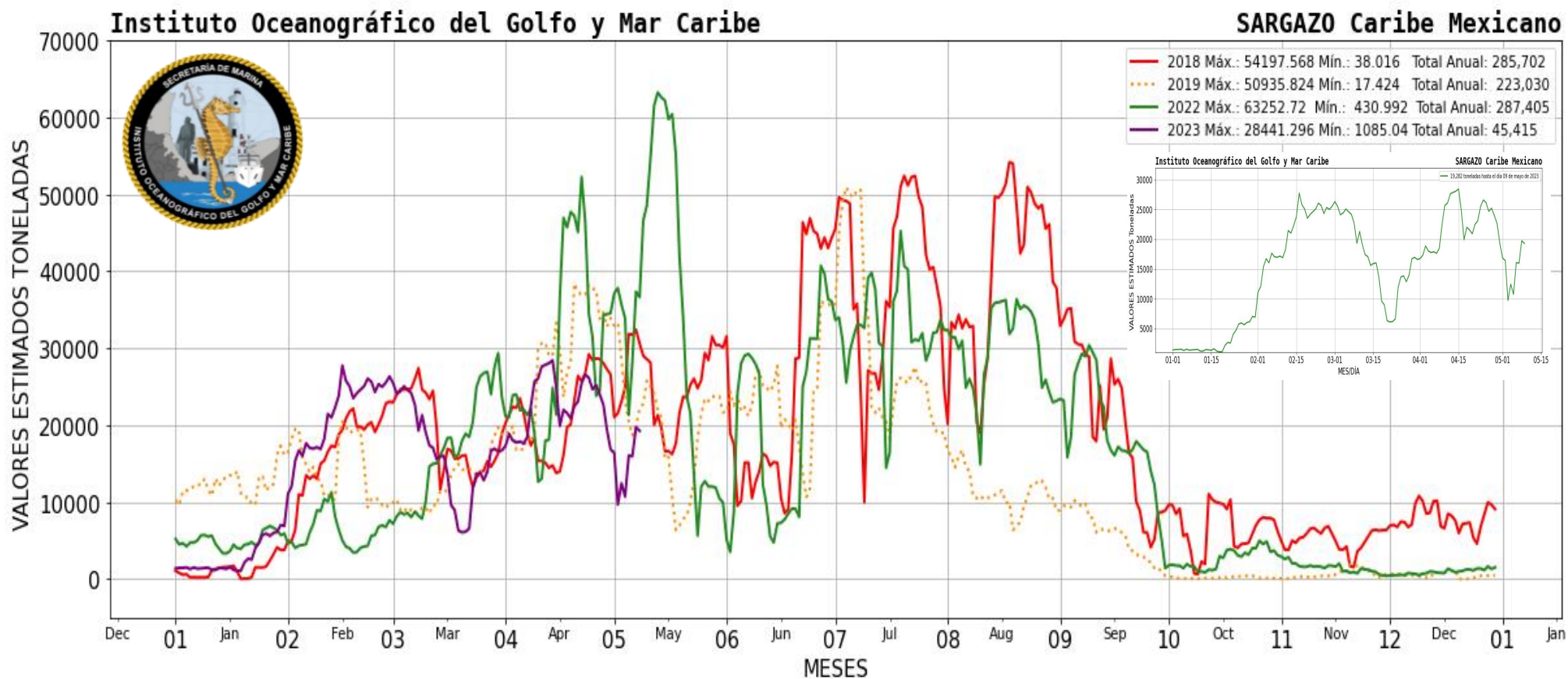
Figura 2.- Presencia aproximada de sargazo en el Caribe Mexicano. Gráfico comparativo de los años 2018, 2019, 2022 y 2023 (gráfico mayor) y valores estimados del 01 de enero al 09 de mayo del presente año (gráfico superior derecha) obtenidos a partir de datos de la USF.
