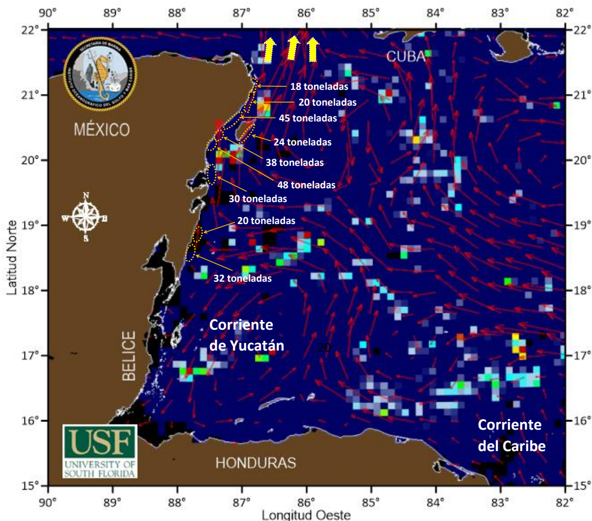
Figura 1.- Cobertura algal ( 09 de mayo ) y modelación de corrientes superficiales ( 10 de mayo ).
