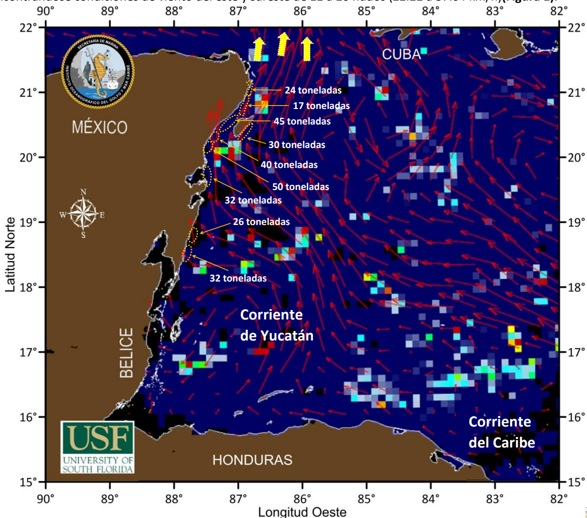
Figura 1.- Cobertura algal ( 12 de mayo ) y modelación de corrientes superficiales ( 13 de mayo ).
