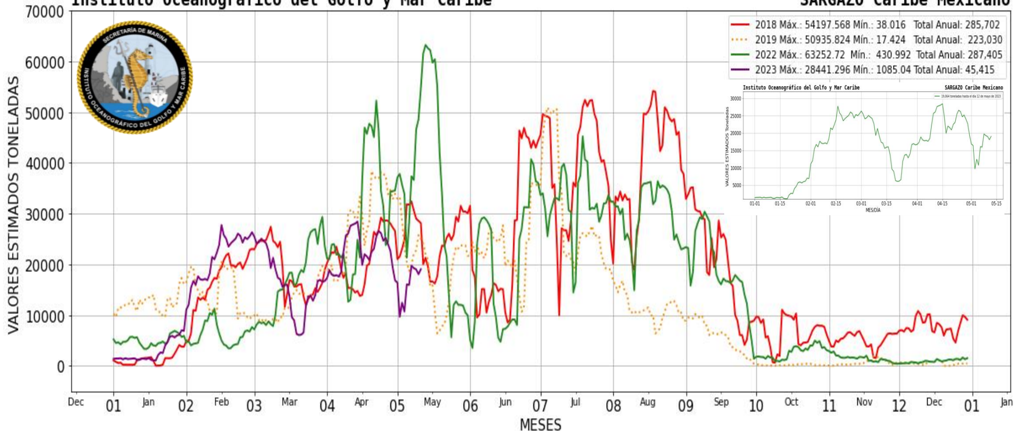
Figura 2.- Presencia aproximada de sargazo en el Caribe Mexicano. Gráfico comparativo de los años 2018, 2019, 2022 y 2023 (gráfico mayor) y valores estimados del 01 de enero al 12 de mayo del presente año (gráfico superior derecha) obtenidos a partir de datos de la USF.
