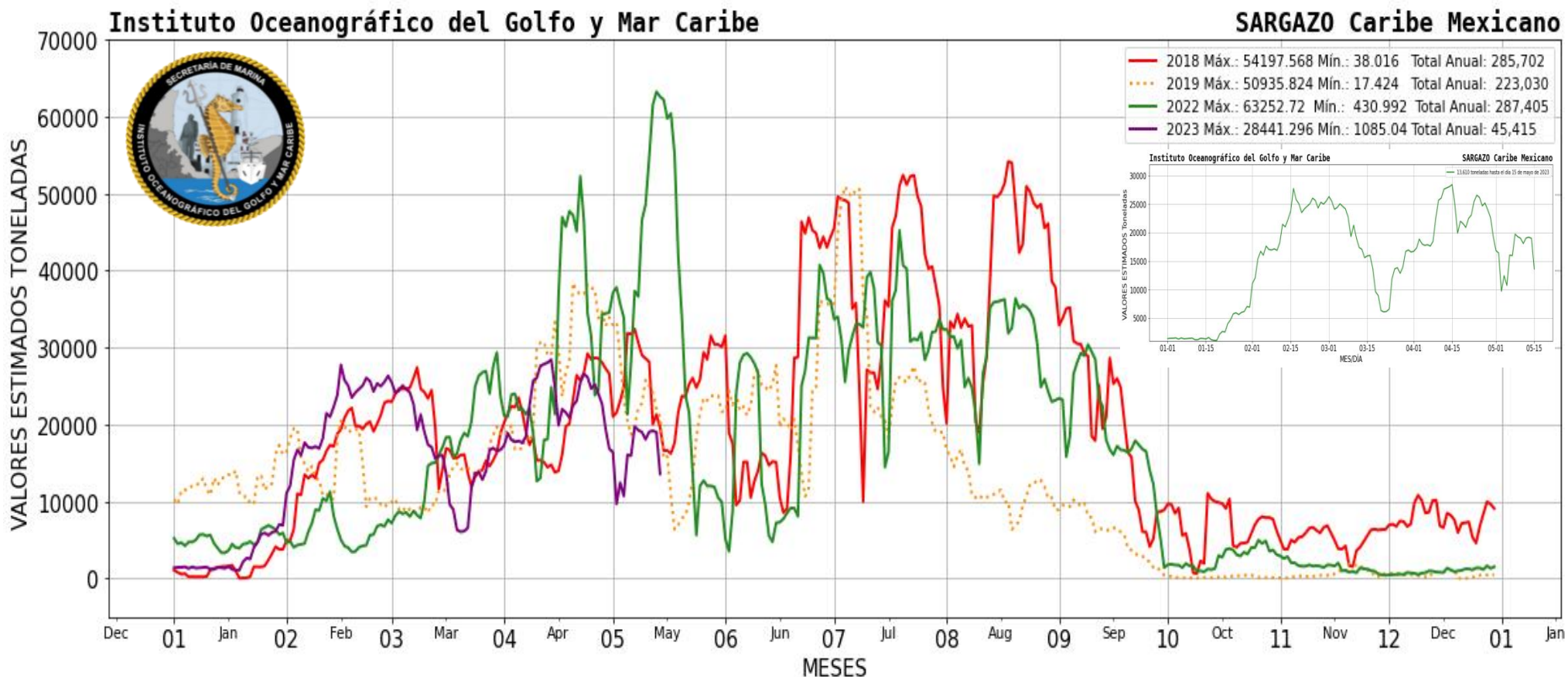
Figura 2.- Presencia aproximada de sargazo en el Caribe Mexicano. Gráfico comparativo de los años 2018, 2019, 2022 y 2023 (gráfico mayor) y valores estimados del 01 de enero al 15 de mayo del presente año (gráfico superior derecha) obtenidos a partir de datos de la USF.
