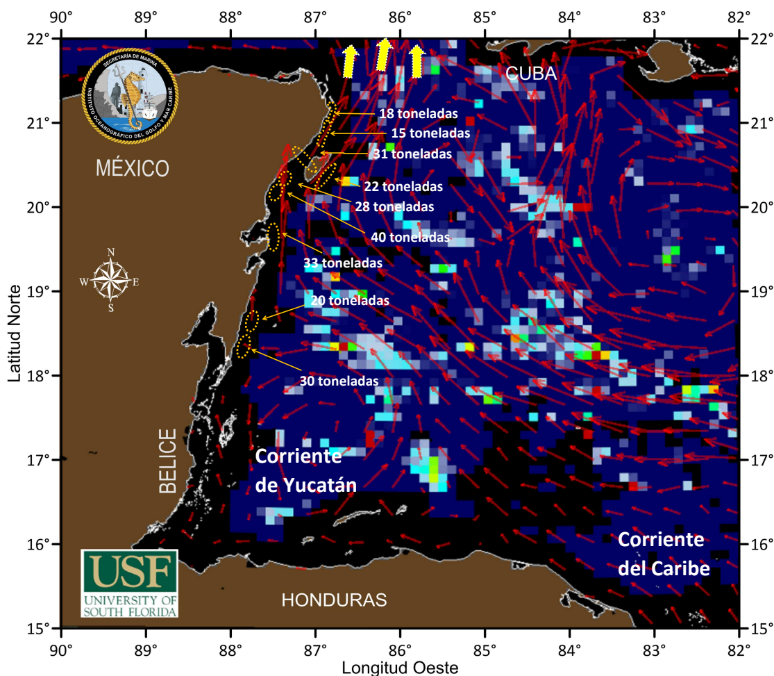
Figura 1.- Cobertura algal ( 15 de mayo ) y modelación de corrientes superficiales ( 16 de mayo ).
