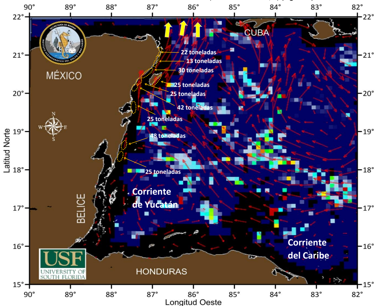
Figura 1.- Cobertura algal ( 17 de mayo ) y modelación de corrientes superficiales ( 18 de mayo ).
