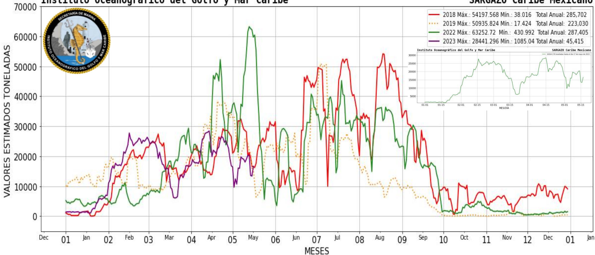
Figura 2.- Presencia aproximada de sargazo en el Caribe Mexicano. Gráfico comparativo de los años 2018, 2019, 2022 y 2023 (gráfico mayor) y valores estimados del 01 de enero al 17 de mayo del presente año (gráfico superior derecha) obtenidos a partir de datos de la USF.
