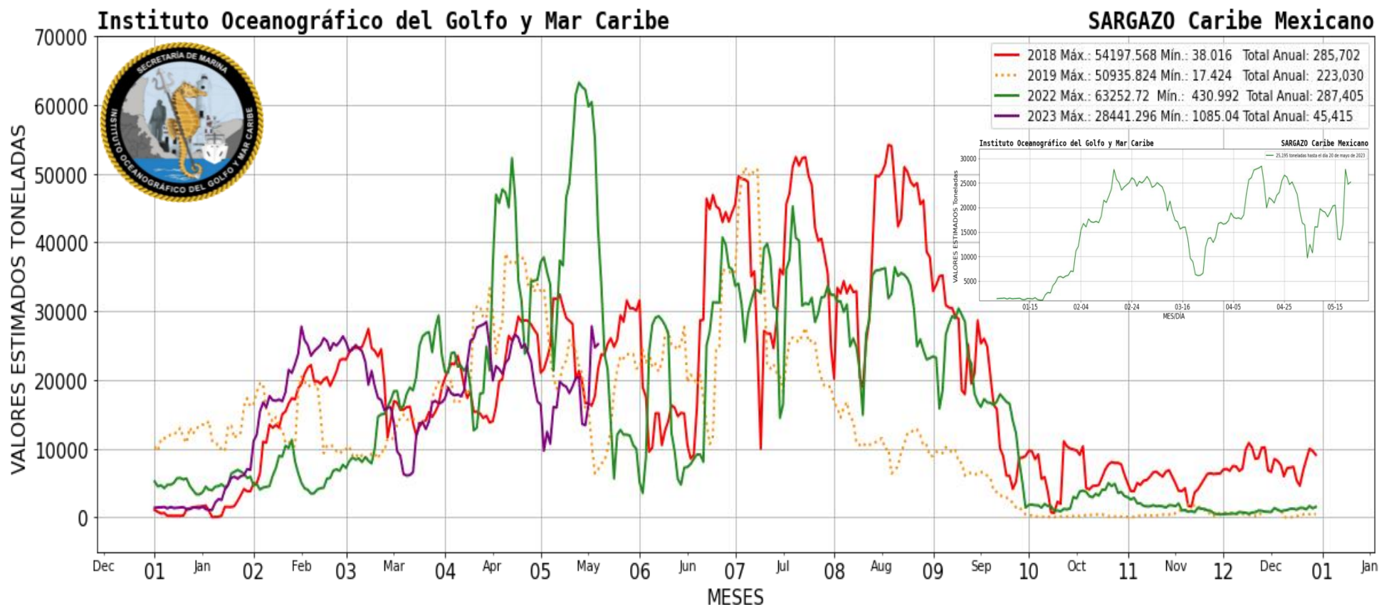
Figura 2.- Presencia aproximada de sargazo en el Caribe Mexicano. Gráfico comparativo de los años 2018, 2019, 2022 y 2023 (gráfico mayor) y valores estimados del 01 de enero al 20 de mayo del presente año (gráfico superior derecha) obtenidos a partir de datos de la USF.
