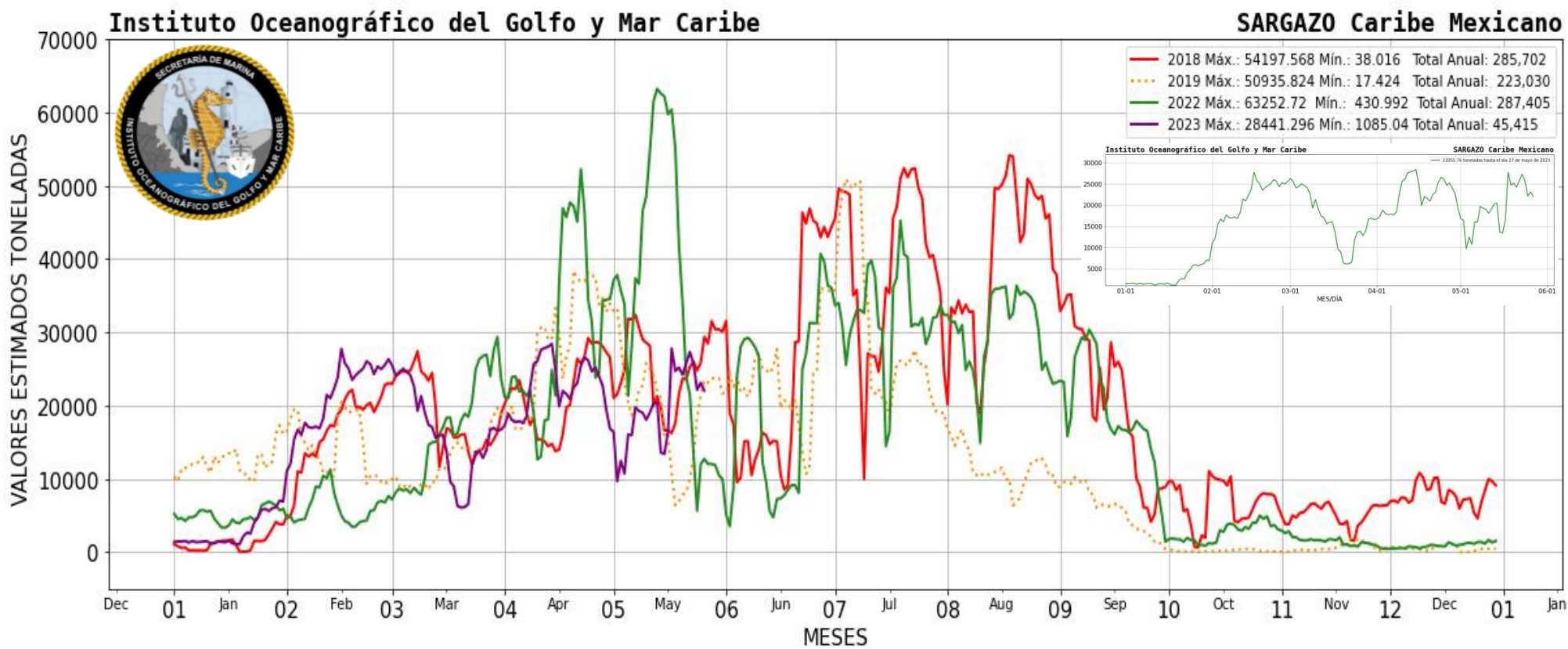
Figura 2.- Presencia aproximada de sargazo en el Caribe Mexicano. Gráfico comparativo de los años 2018, 2019, 2022 y 2023 (gráfico mayor) y valores estimados del 01 de enero al 27 de mayo del presente año (gráfico superior derecha) obtenidos a partir de datos de la USF.
