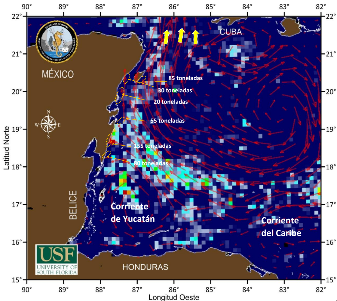
Figura 1.- Cobertura algal ( 27 de mayo ) y modelación de corrientes superficiales ( 28 de mayo ).
