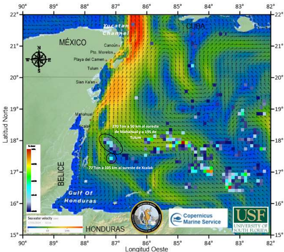
Figura 2.- Cobertura algal (16 de mayo) y la modelación de corrientes superficiales (17 de mayo), obtenidos a partir de datos de la USF.
