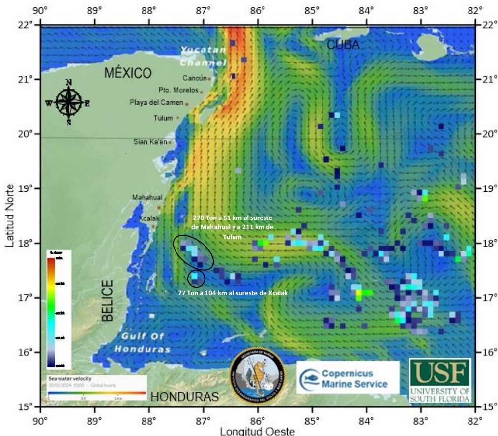
Figura 2.- Cobertura algal (19 de mayo) y la modelación de corrientes superficiales (20 de mayo), obtenidos a partir de datos de la USF.
