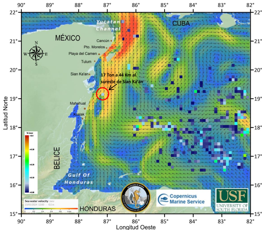
Figura 2.- Cobertura algal (22 de mayo) y la modelación de corrientes superficiales (23 de mayo), obtenidos a partir de datos de la USF.
