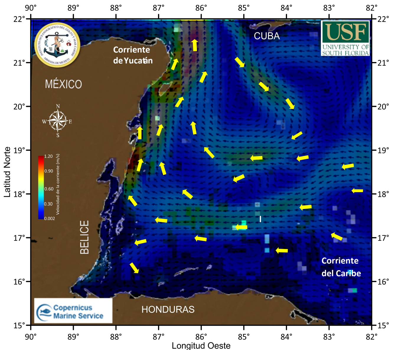
Figura 1.- Cobertura algal (06 de octubre) y modelación de corrientes superficiales (07 de octubre).
