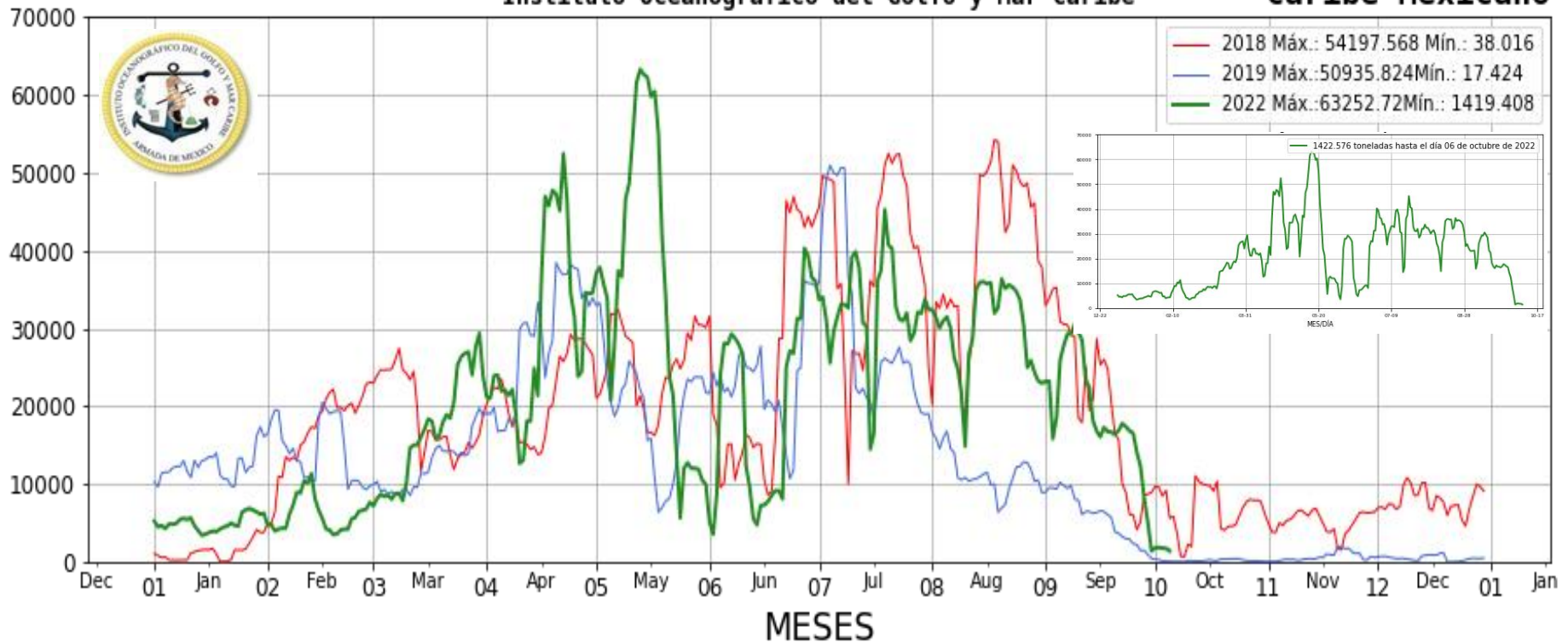
Figura 2.- Valores estimados de la cantidad de sargazo en el Caribe Mexicano. Gráfico comparativo de los años 2018, 2019 y 2022 (gráfico mayor) y valores estimados del 01 de enero al 06 de octubre del presente año (gráfico superior derecha) obtenidos a partir de datos de la USF.
