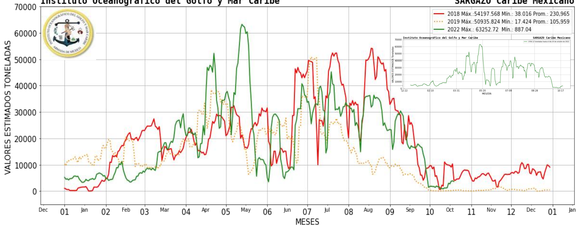
Figura 2.- Valores estimados de la cantidad de sargazo en el Caribe Mexicano. Gráfico comparativo de los años 2018, 2019 y 2022 (gráfico mayor) y valores estimados del 01 de enero al 20 de octubre del presente año (gráfico superior derecha) obtenidos a partir de datos de la USF.
