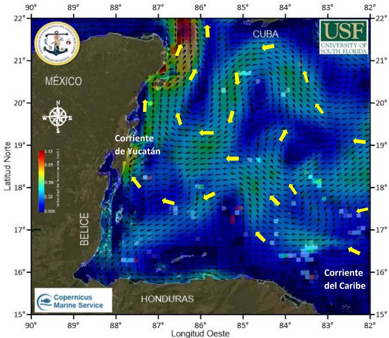
Figura 1.- Cobertura algal (20 de octubre) y modelación de corrientes superficiales (21 de octubre).
