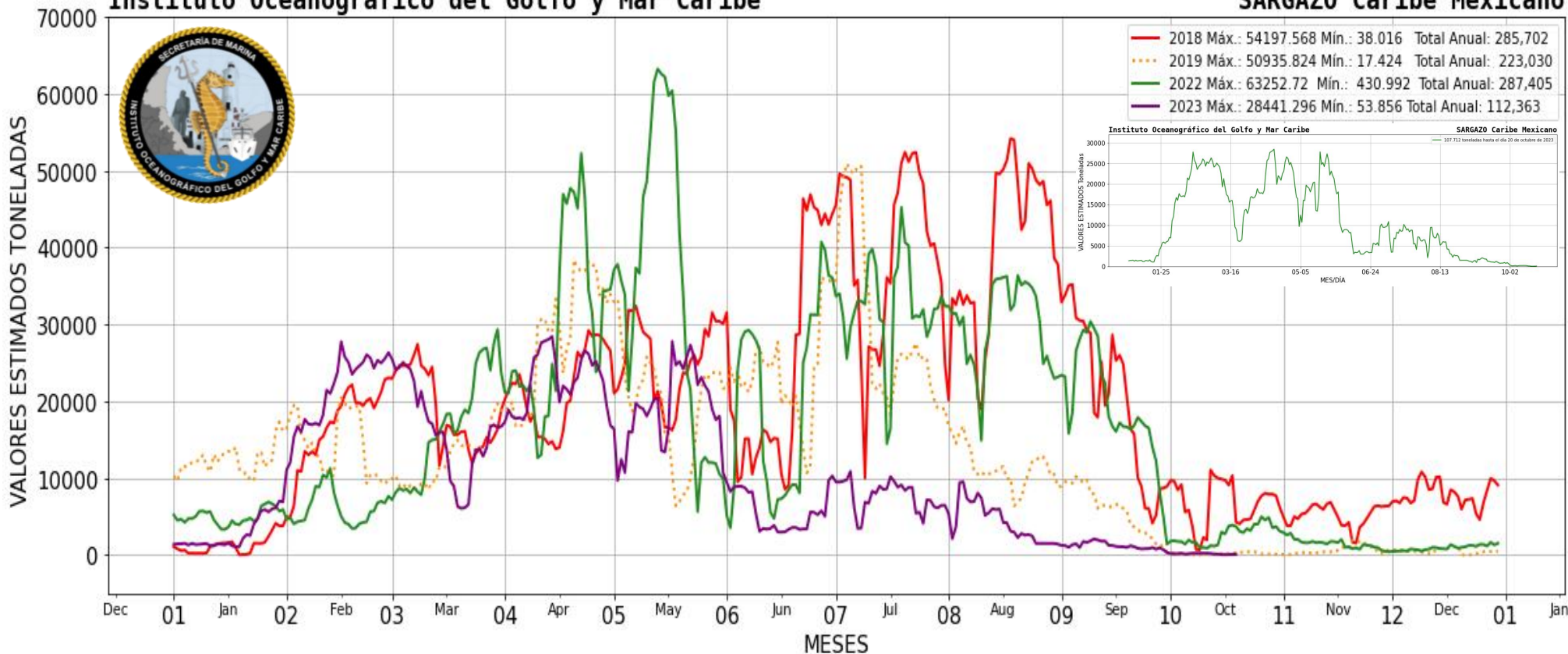
Figura 2.- Presencia aproximada de sargazo en el Caribe Mexicano. Gráfico comparativo de los años 2018, 2019, 2022 y 2023 (gráfico mayor) y valores estimados del 01 de enero al 20 de octubre del presente año (gráfico superior derecho) obtenidos a partir de datos de la USF.
