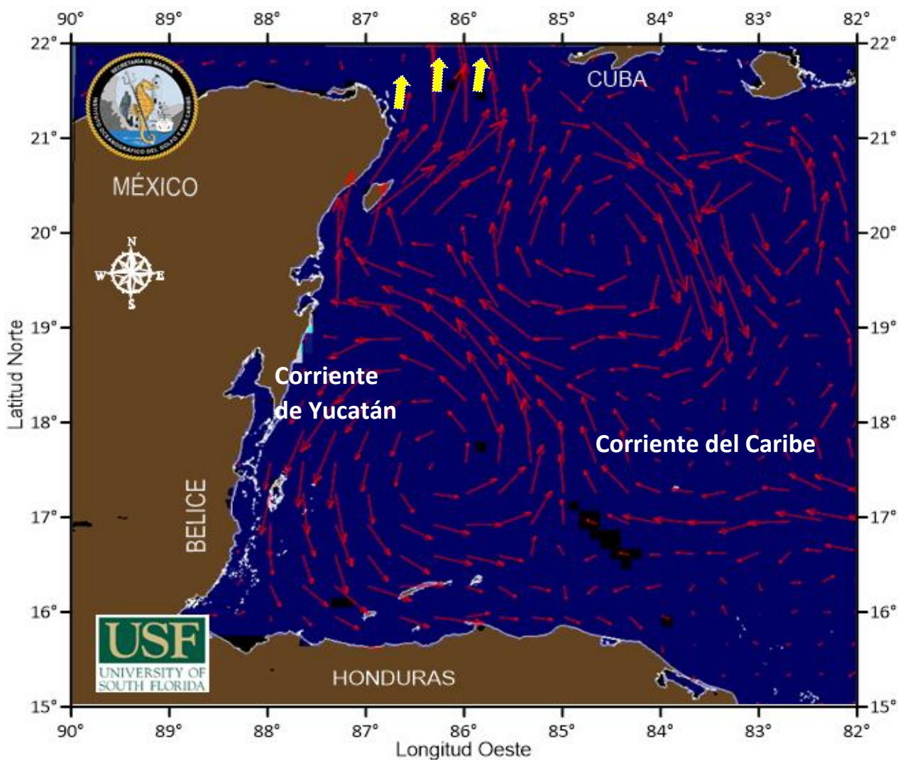
Figura 1.-Cobertura algal (20 de octubre) y la modelación de corrientes superficiales (21 de octubre), obtenidos a partir de datos de la USF.
